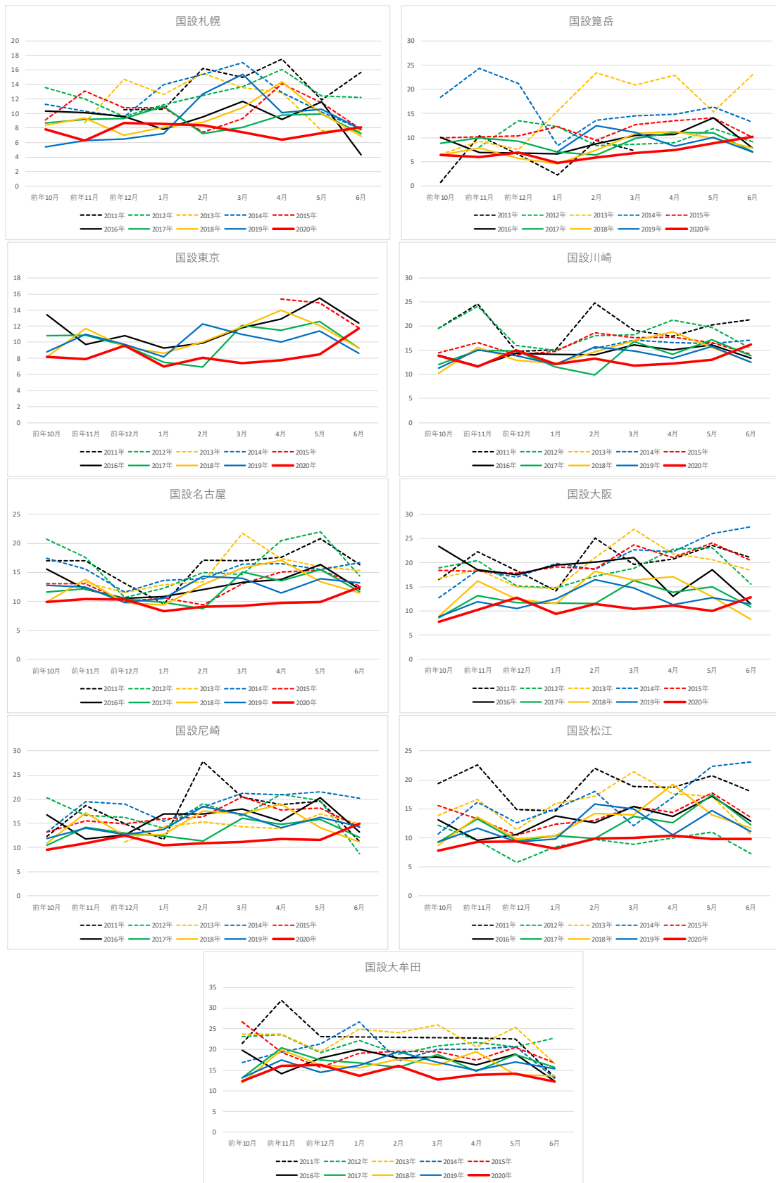
図1 国設大気測定局ごとの2011年～2020年におけるPM2.5濃度の推移
