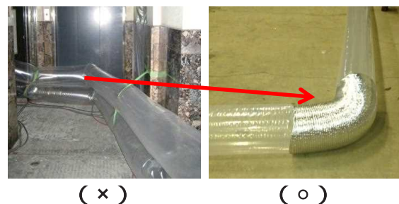
図 3. 53. 1 排気ダクトの例
