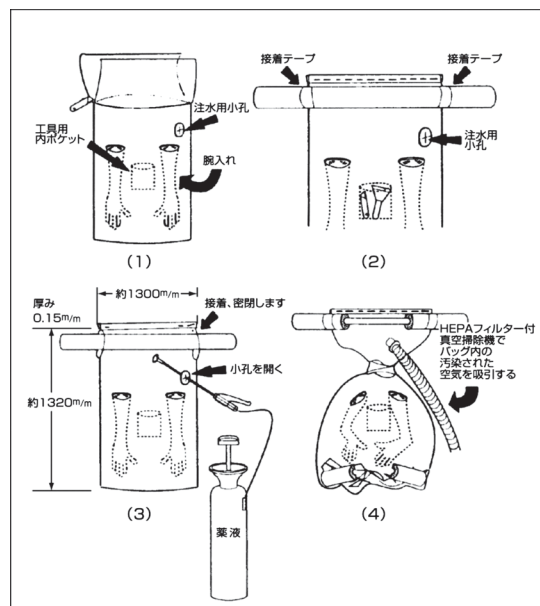
図 3.86 グローブバッグの例
