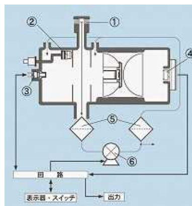
図 3. 130 粉じん相対濃度計の構造の例
