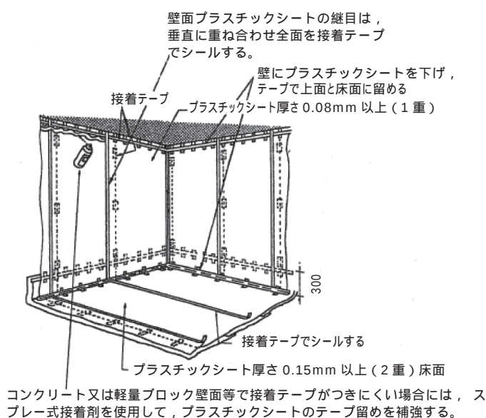
図 3. 21 壁面の隔離養生例
