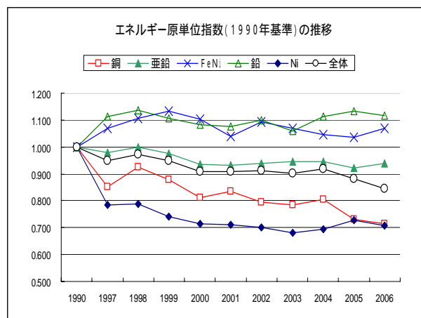
図2. エネルギー原単位指数の推移
