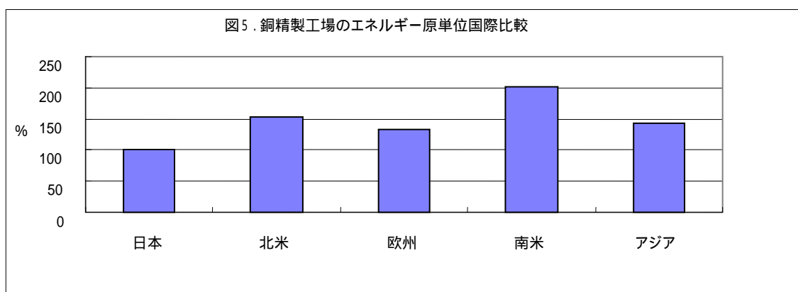
図5 . に銅精製工場（電解工場）のエネルギー原単位の国際比較を示す。
