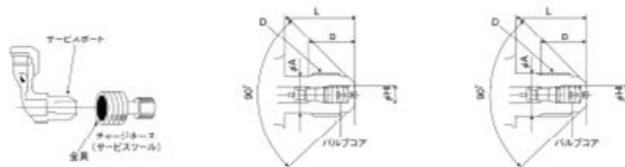
接続図
