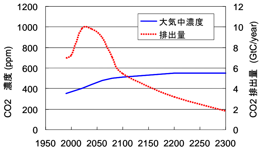
図-2.4 550ppm 安定化経路の例
