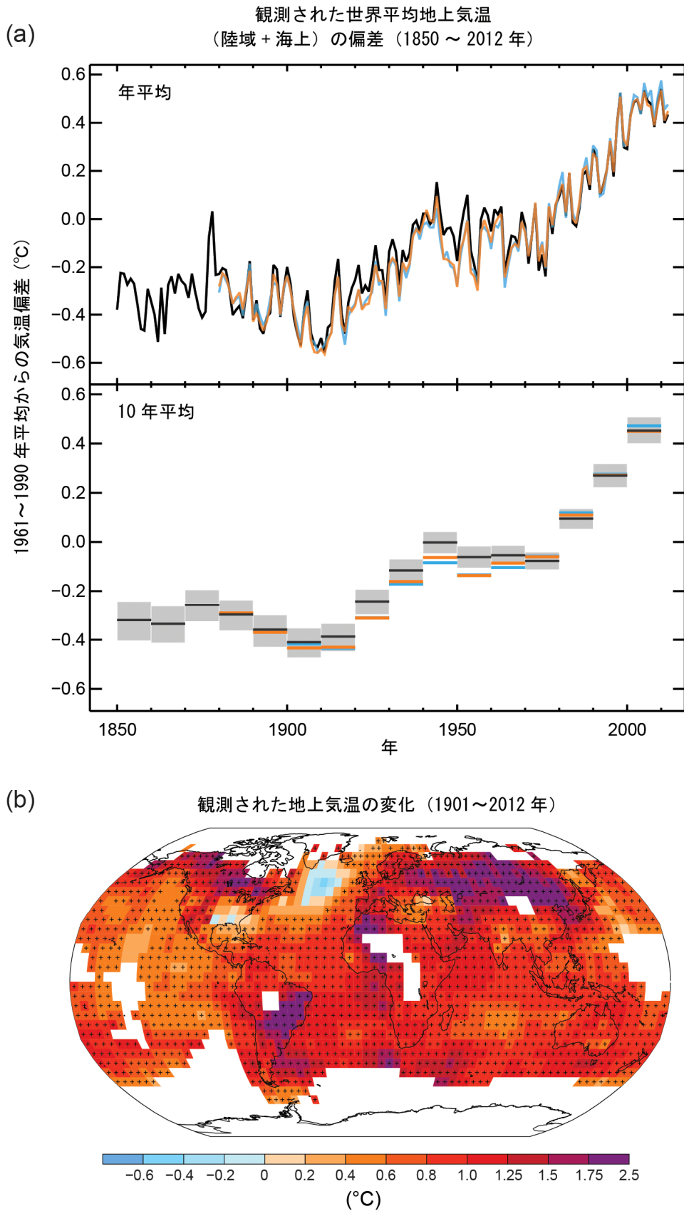
図 SPM.1: (a) 3つのデータセットによる、1850年から2012年までに観測された陸域と海上とを合わせた世界平均地上気温の偏差。上図: 年平均値、下図: 10年ごとの平均値(黒色のデータセットについては不確実性の推定を含む)。1961~1990年平均からの偏差。(b) 図 a のオレンジ色のデータセットから線形回帰で求めた気温の変化傾向による1901年から2012年の地上気温変化の分布。変化傾向は、データが有効で確実な推定が可能である場所(すなわち、70%以上の完全な記録がそろっており、かつ期間の最初の10%と最後の10%においてそれぞれ20%以上のデータが利用可能な格子のみ)について計算されている。それ以外の領域は白色としている。危険率10%の水準で変化傾向が有意である格子点を+の記号で示す。データセットの一覧と、更に詳細な技術情報は、技術要約の補足資料を参照。{図 2.19~2.21、図 TS.2}
