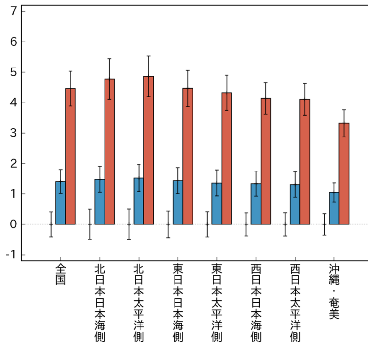
図 2-5 気象庁の予測による年平均気温の将来変化 (°C)
