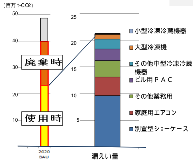
図3: 2020年排出予測に占める使用時漏えい
