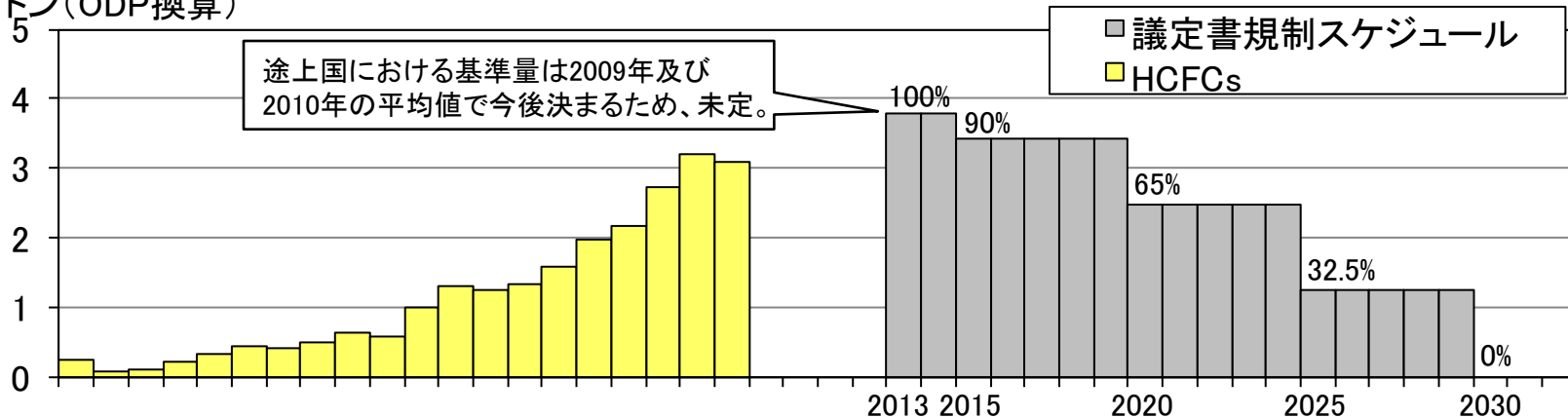
モントリオール議定書に基づくCFCs及びHCFCs消費量の推移(途上国の合計)
