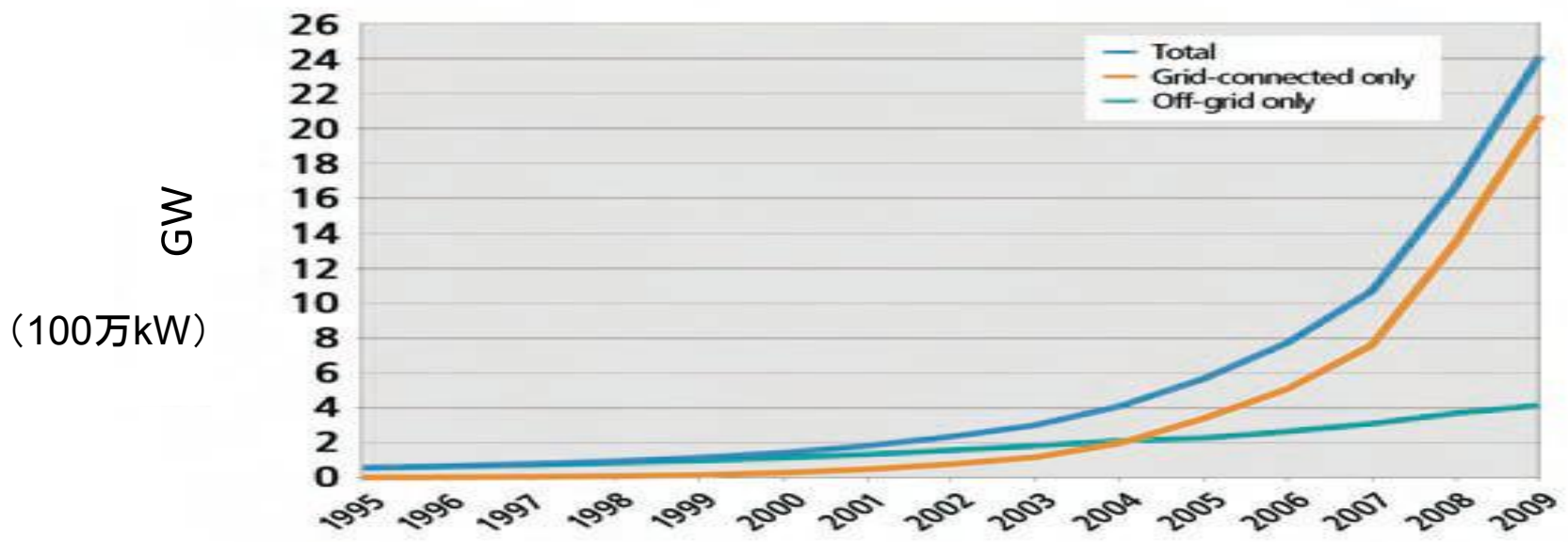
世界の太陽光発電容量の推移(累積、1995～2009)
