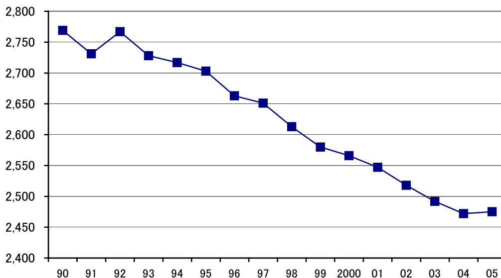
図-3 セメント製造用熱エネルギー原単位の推移 (MJ/t-セメント) (エネルギー代替廃棄物等を含まず)
