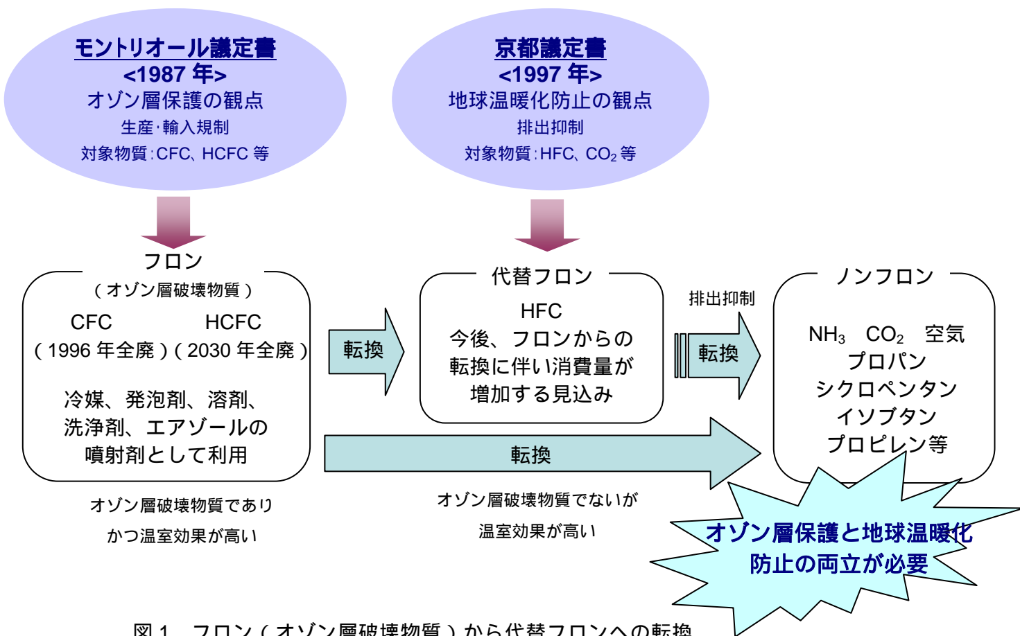
図1 フロン（オゾン層破壊物質）から代替フロンへの転換
