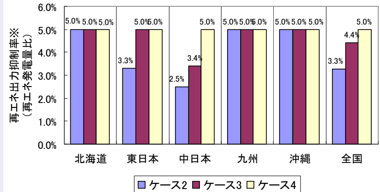
蓄電池導入時における出力抑制必要量
