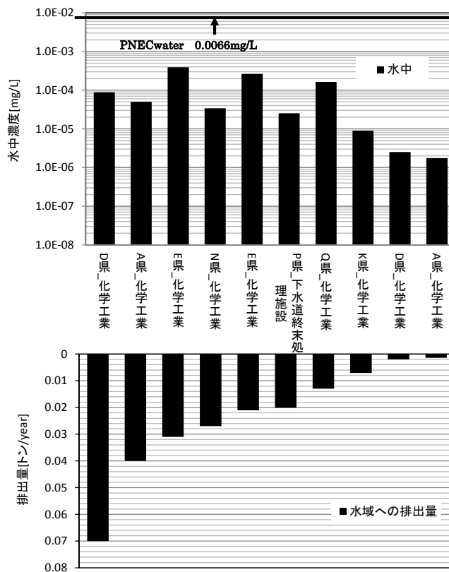
7 8 9 図 5-5 PRTR 届出事業所毎の排出量に対する水中濃度
