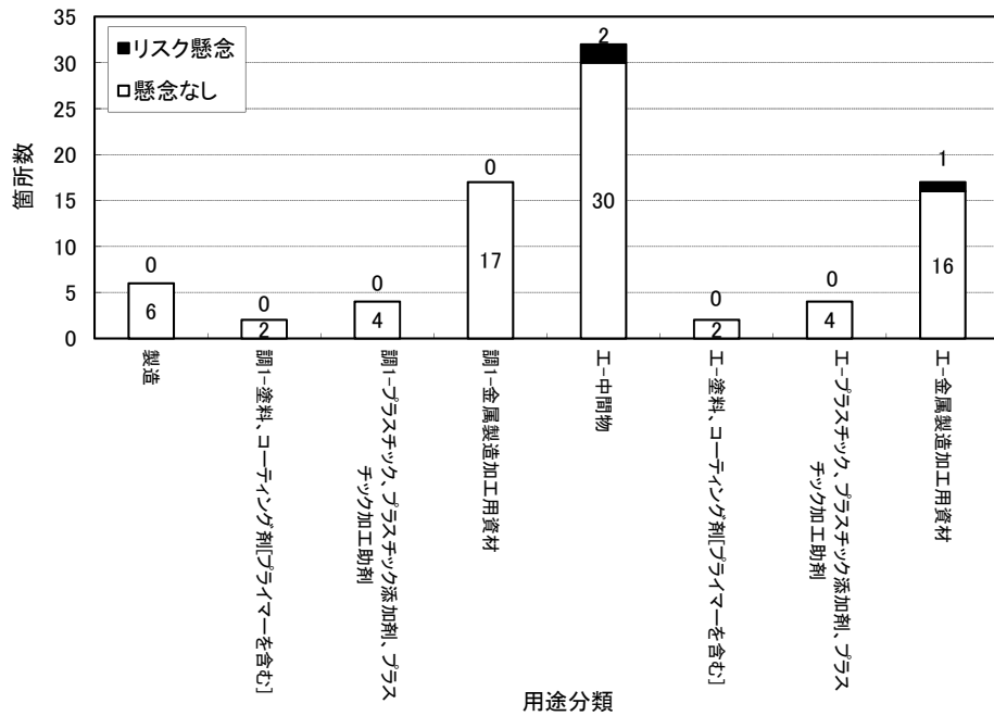
9 10 図 5-4 化審法届出情報に基づく仮想的な排出源(水域)の用途別リスク懸念箇所数
