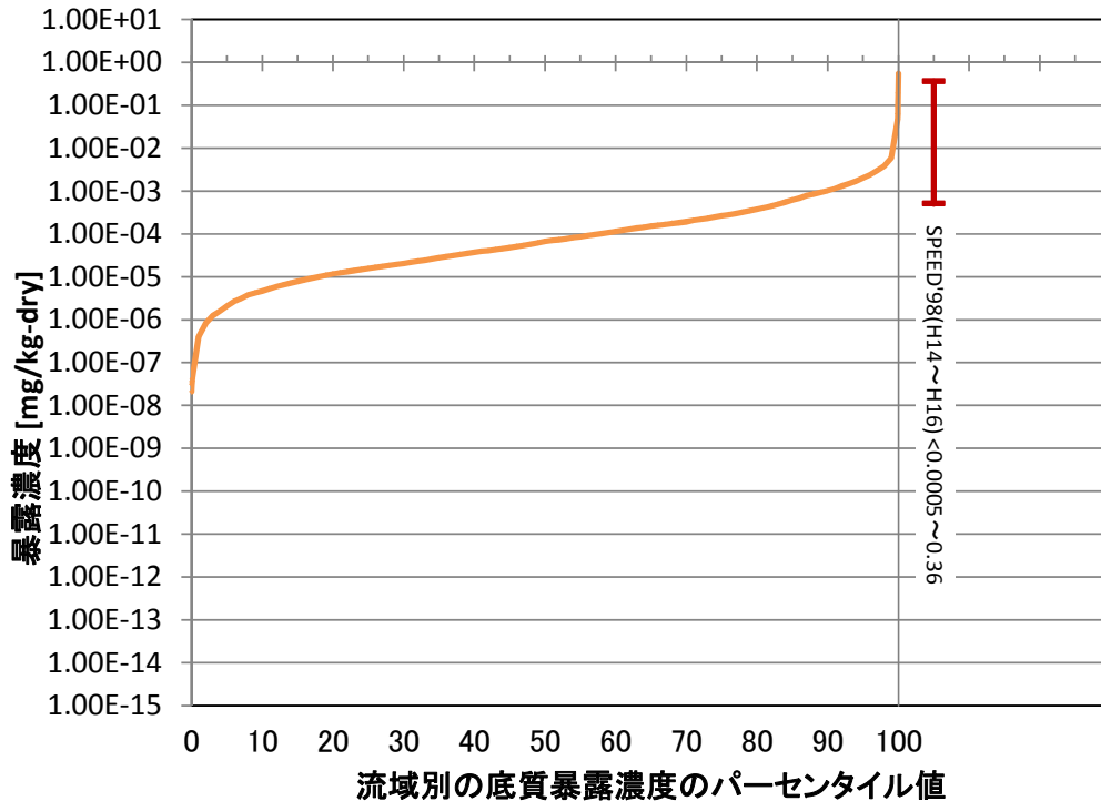
図 5-11 G-CIEMS 推計濃度とモニタリング濃度の範囲の比較(底質)
