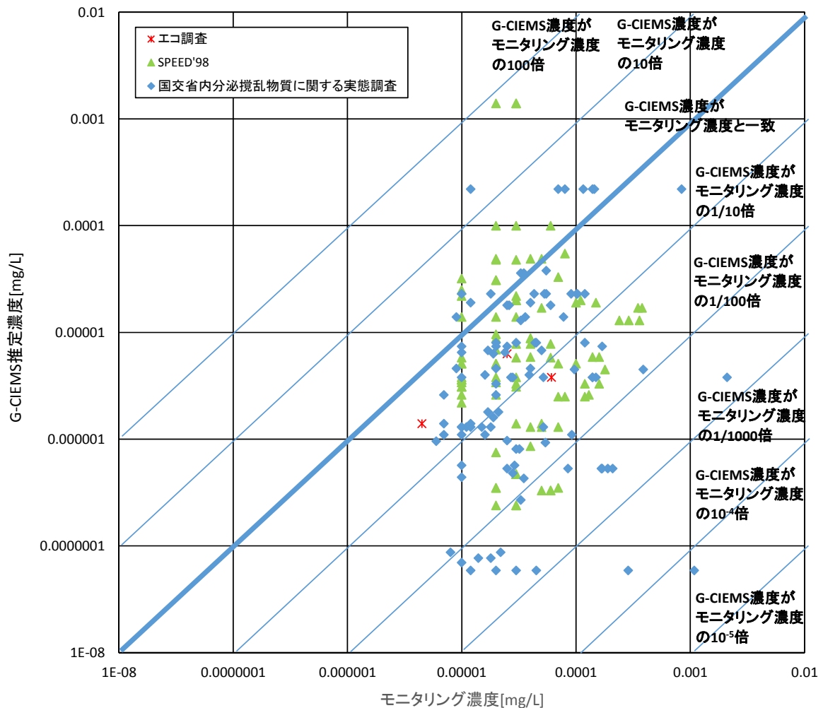
13 14 図 7-1 環境基準点を含む流域における G-CIEMS 推計水質濃度とモニタリング水質濃度 15 の比較 (SPEED'98(平成 14~16 年度)、エコ調査(平成 17 年度)、国土交通省全国一級河川 16 における内分分泌攪乱物質に関する実態調査 (平成 14~23 年度))
