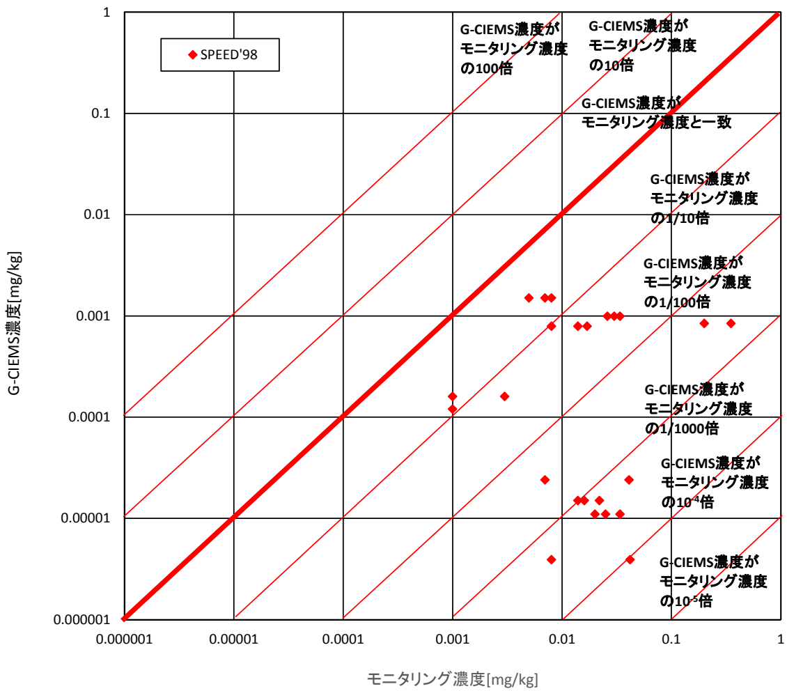
1 2 図 7-2 環境基準点を含む流域における G-CIEMS 推定底質濃度とモニタリング底質濃度 3 の比較 (SPEED'98(平成 14~16 年度)) 4 5
