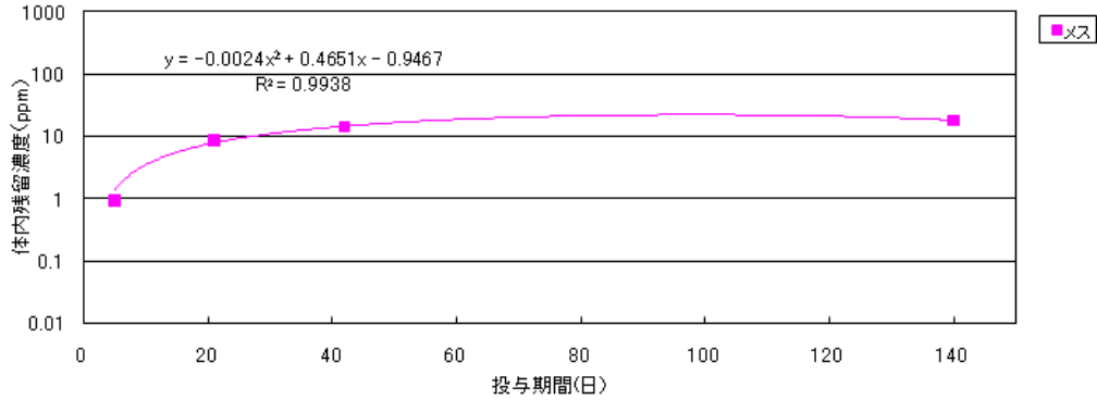
図 4 p,p' -DDT25ppm添加飼料の給与期間とウズラ体内の p,p' -DDE残留濃度の関係
