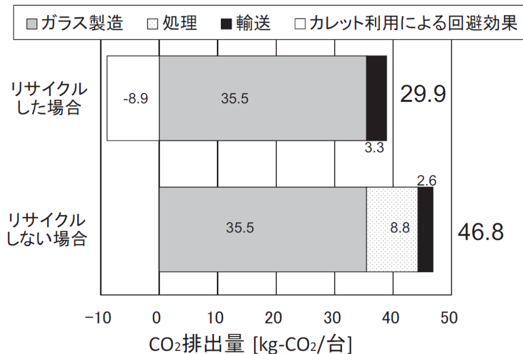
ELVからの板ガラスリサイクルシステムのLCA結果
