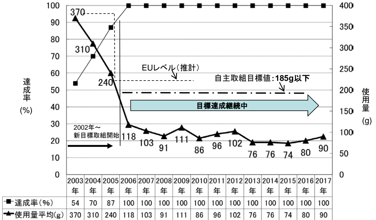
図1. 鉛使用量削減状況(乗用車平均)2003年～2017年(1～12月)推移
