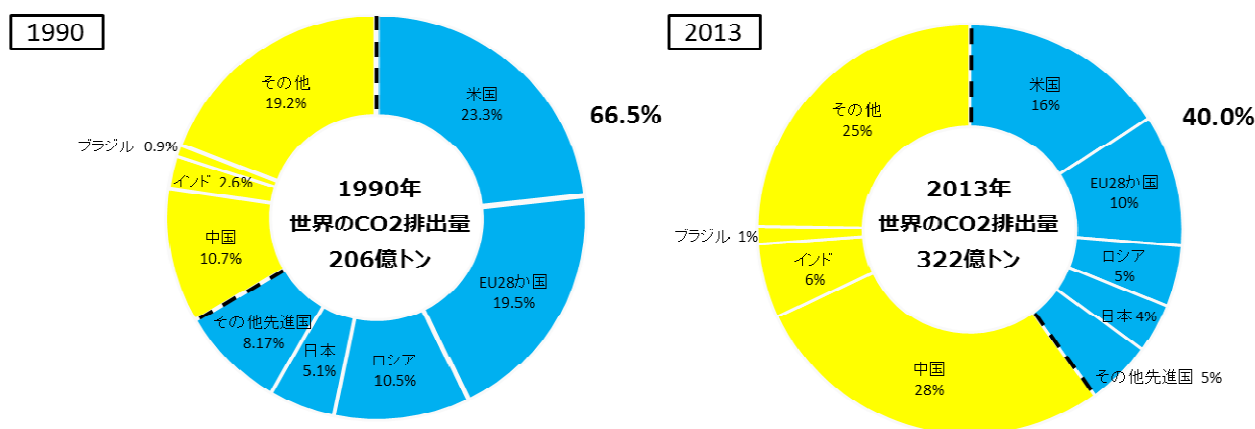
図表 - 4 - 3 . 世界のエネルギー起源CO 2 排出量グラフ （附属書 国と非附属書 国との比較）
