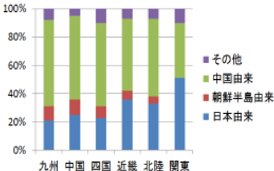
図表Ⅲ－5－19. PM 2.5 の国内及び国外の寄与割合(2010年通年を対象とした推計例)
