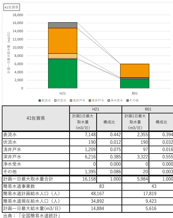
図 5-7 水源種別毎の計画一日最大取水量の推移(都道府県別、簡易水道事業)(11)
