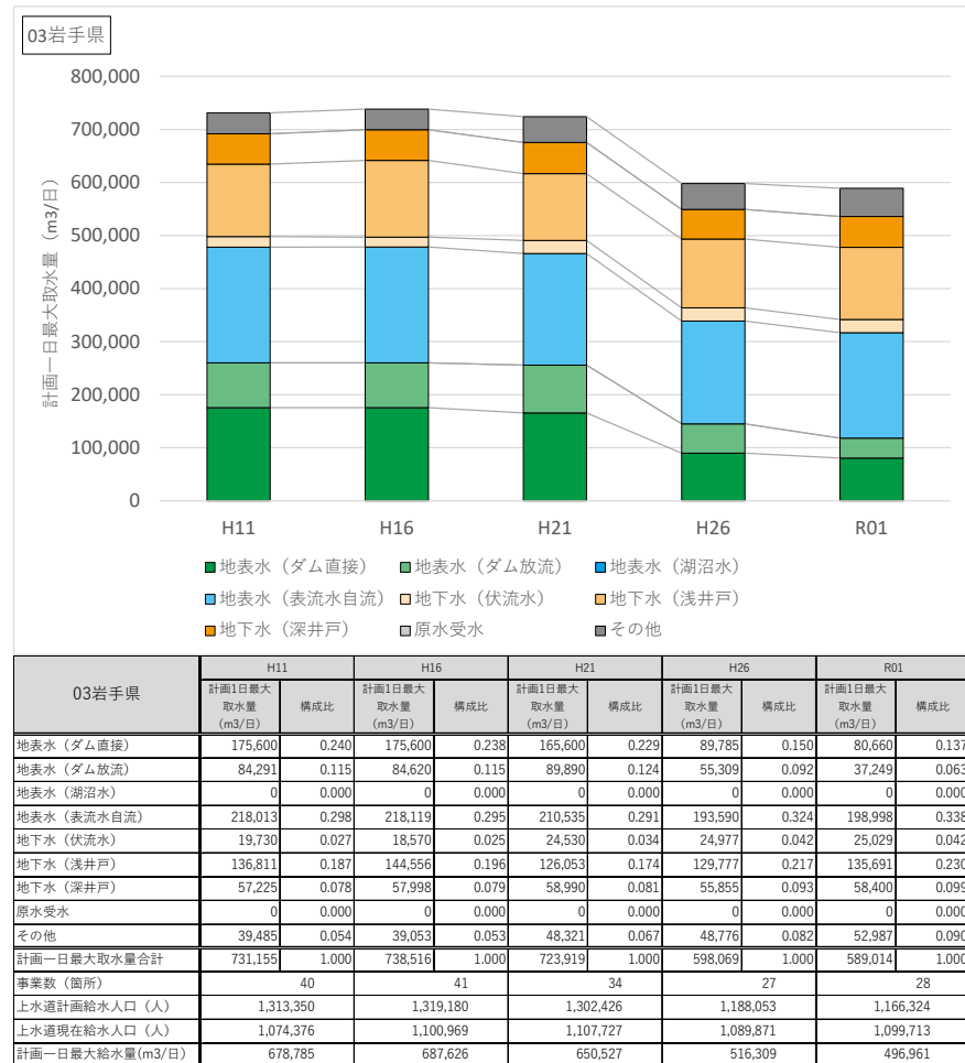
図 5-3 水源種別毎の計画一日最大取水量の推移(上水道事業と水道用水供給事業)(2)
