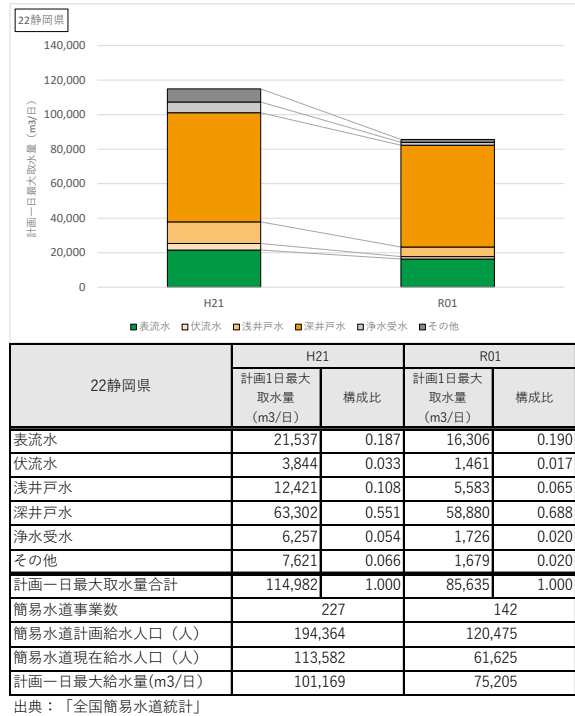
図 5-7 水源種別毎の計画一日最大取水量の推移(都道府県別、簡易水道事業)(6)
