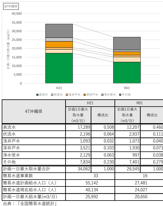
図 5-7 水源種別毎の計画一日最大取水量の推移(都道府県別、簡易水道事業)(13)
