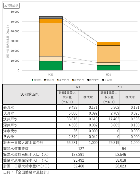
図 5-7 水源種別毎の計画一日最大取水量の推移(都道府県別、簡易水道事業)(8)
