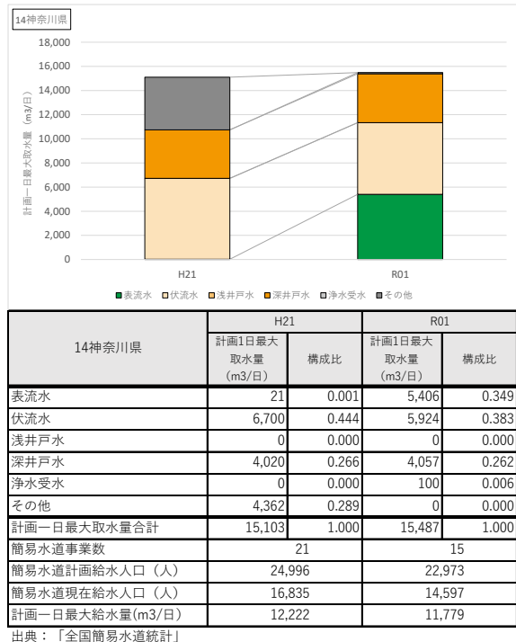
図 5-7 水源種別毎の計画一日最大取水量の推移(都道府県別、簡易水道事業)(4)
