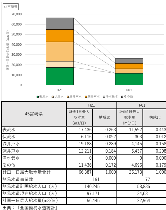
図 5-7 水源種別毎の計画一日最大取水量の推移(都道府県別、簡易水道事業)(12)
