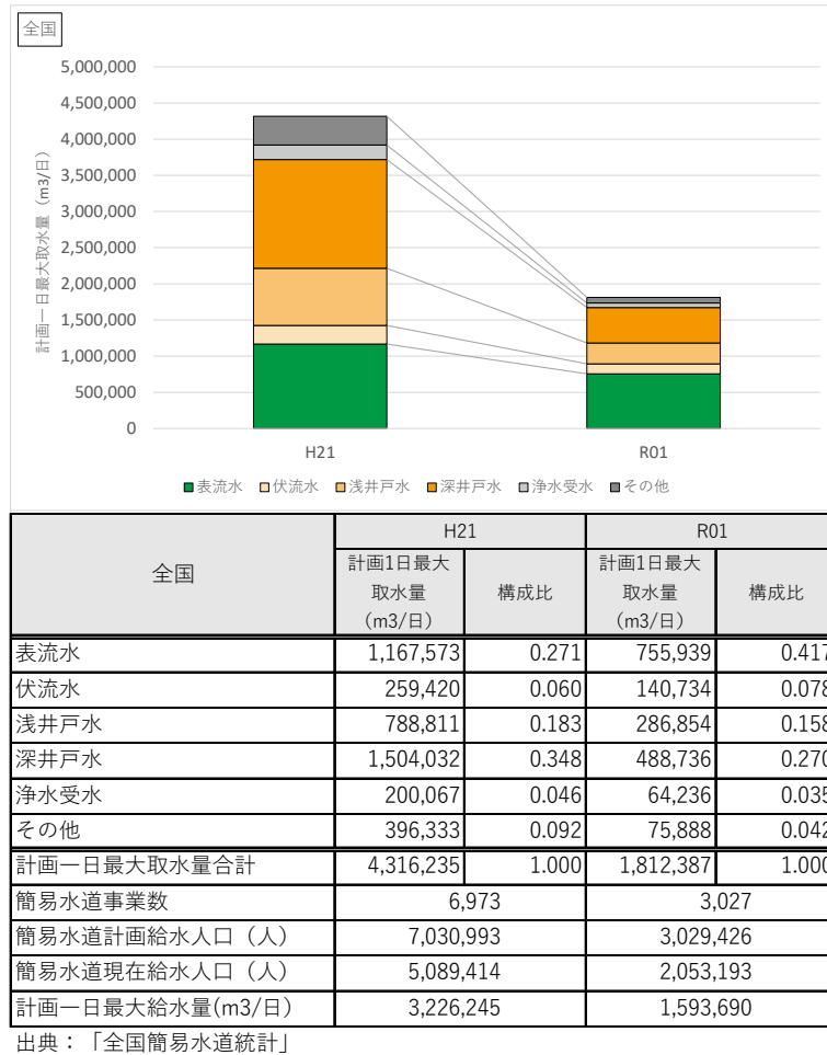
図 5-6 水源種別毎の計画一日最大取水量の推移(全国、簡易水道事業)
