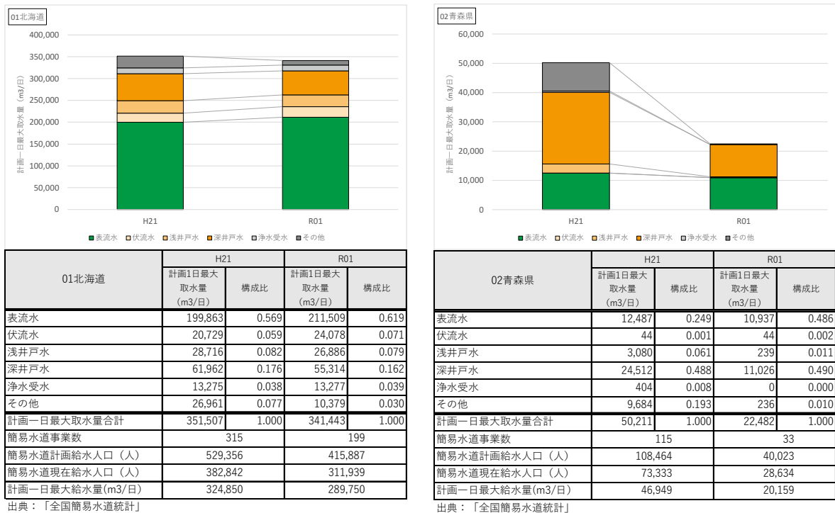
図 5-7 水源種別毎の計画一日最大取水量の推移(都道府県別、簡易水道事業)(1)
