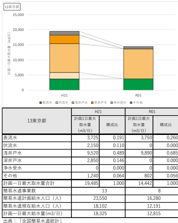
図 5-7 水源種別毎の計画一日最大取水量の推移(都道府県別、簡易水道事業)(4)
