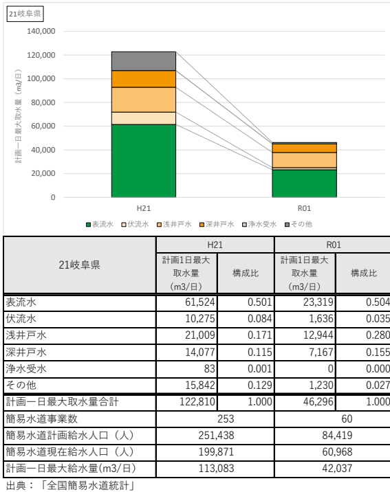
図 5-7 水源種別毎の計画一日最大取水量の推移(都道府県別、簡易水道事業)(6)
