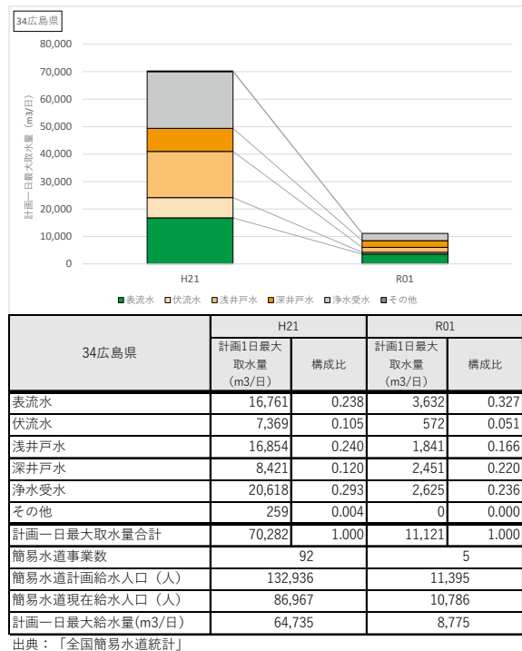
図 5-7 水源種別毎の計画一日最大取水量の推移(都道府県別、簡易水道事業)(9)
