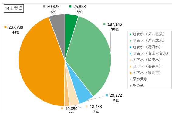
図 5-2 水源種別構成(都道府県別、上水道事業と水道用水供給事業)(3)
