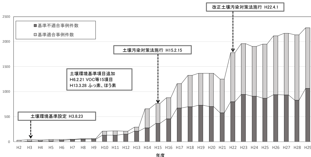
図 6-1 年度別の土壌汚染調査事例
