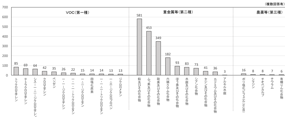
図 6-2 特定有害物質別の基準不適合事例数 (平成 29 年度)
