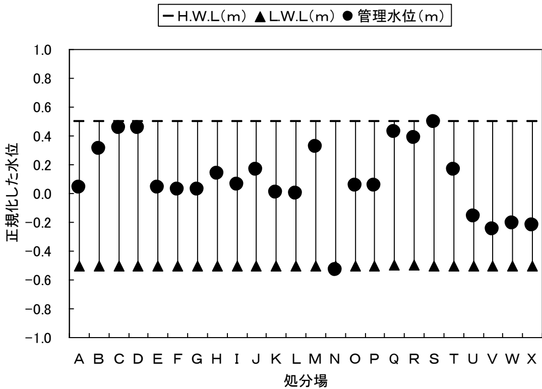
図 A1-2-2 既存海面最終処分場の管理水位 （平成 22 年度調査：HWL と LWL を用いて正規化した水位）
