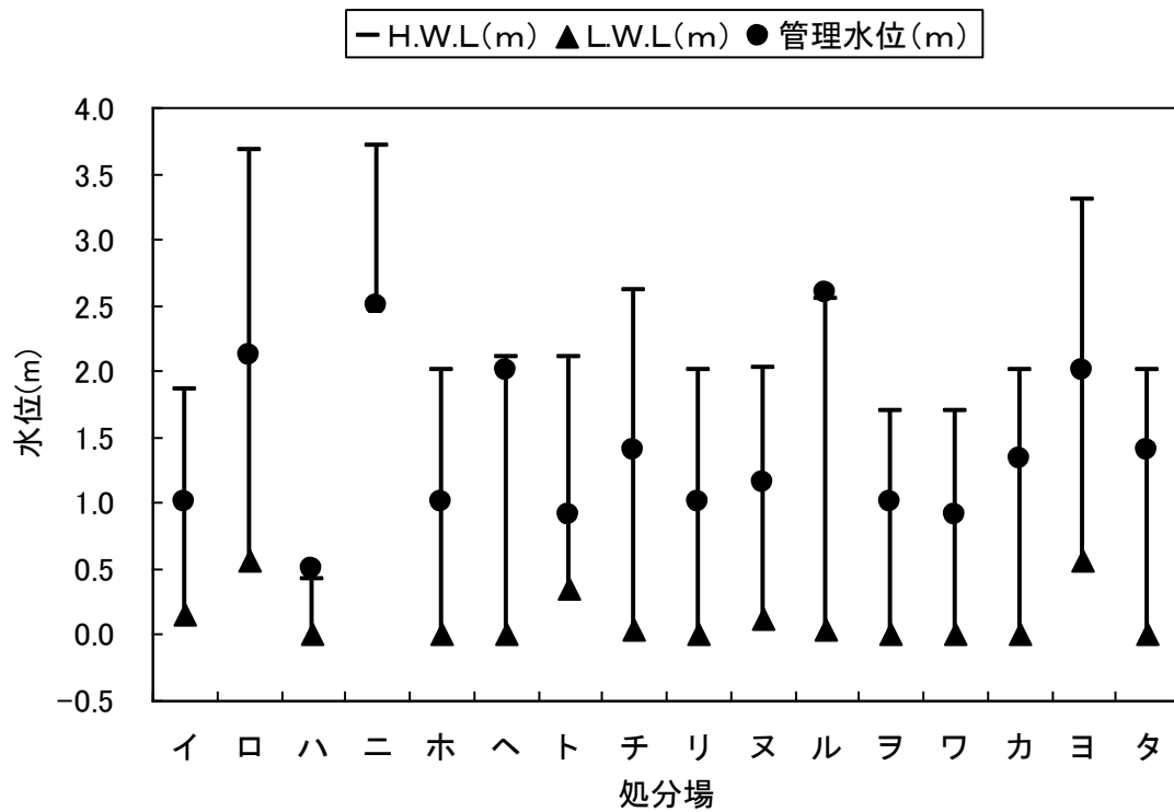
図 A1-1-1 既存海面最終処分場の管理水位（平成 17 年度調査：実際の水位）
