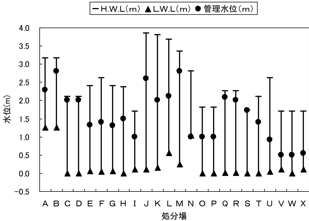
図 A1-2-1 既存海面最終処分場の管理水位（平成 22 年度調査：実際の水位）
