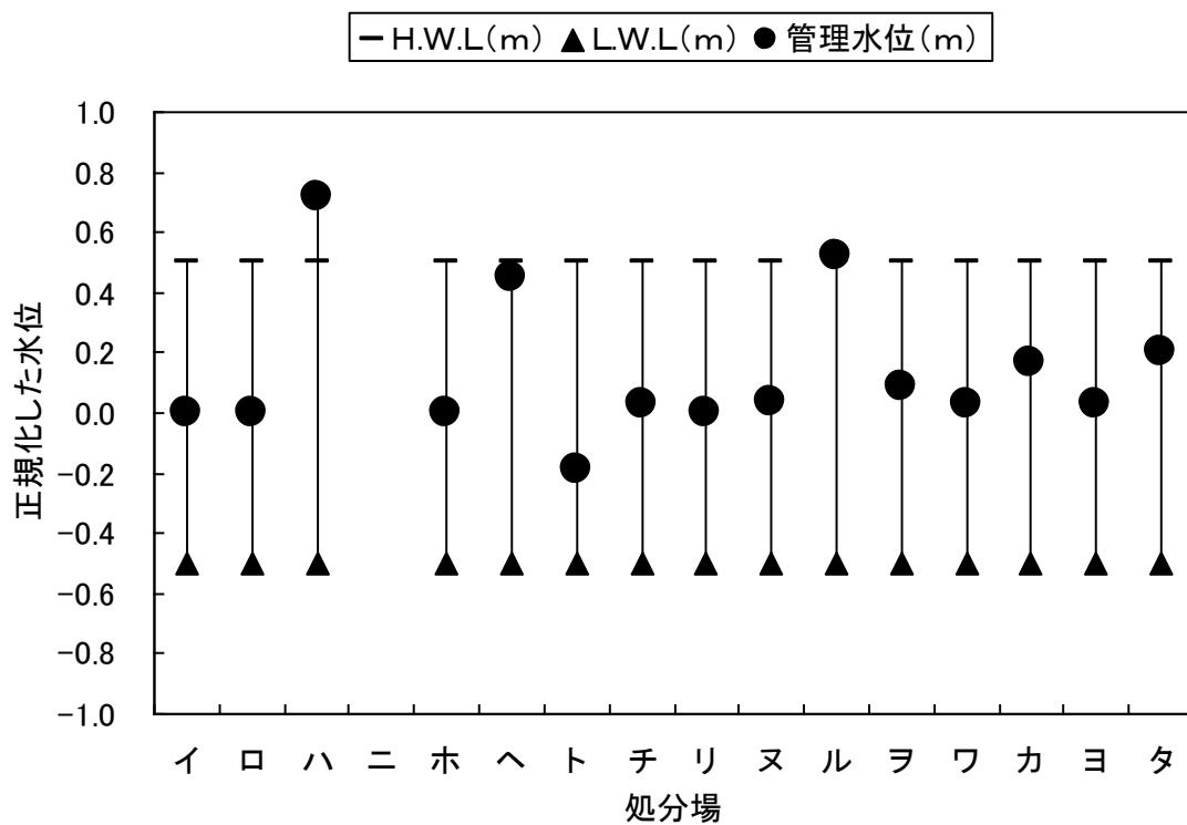
図 A1-1-2 既存海面最終処分場の管理水位 （平成 17 年度調査：HWL と LWL を用いて正規化した水位）
