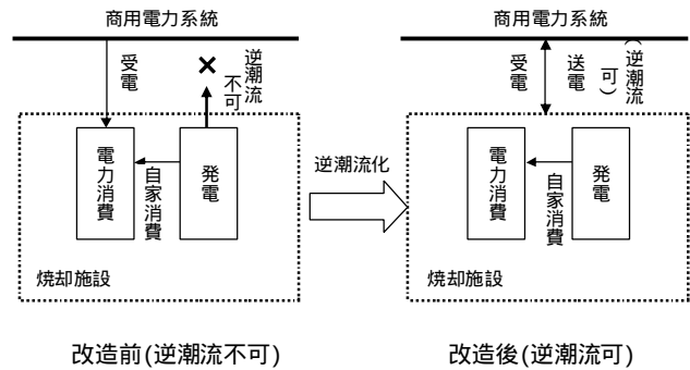
逆潮流化への改造イメージ
