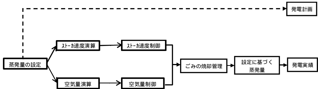
ストーク式焼却炉における自動燃焼制御の例
