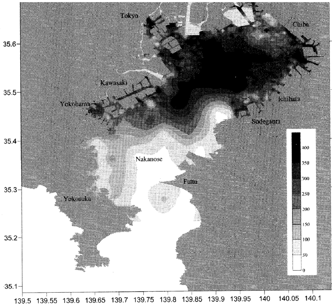
図 1.1.52 東京湾の含水比の分布
