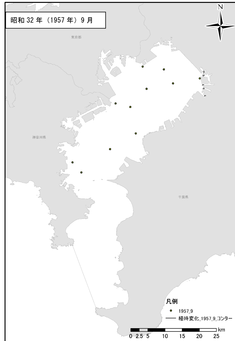
図 1.1.42(3) 昭和 30 年（1955 年）～昭和 44 年（1969 年）の東京湾の底層溶存酸素量の状況
