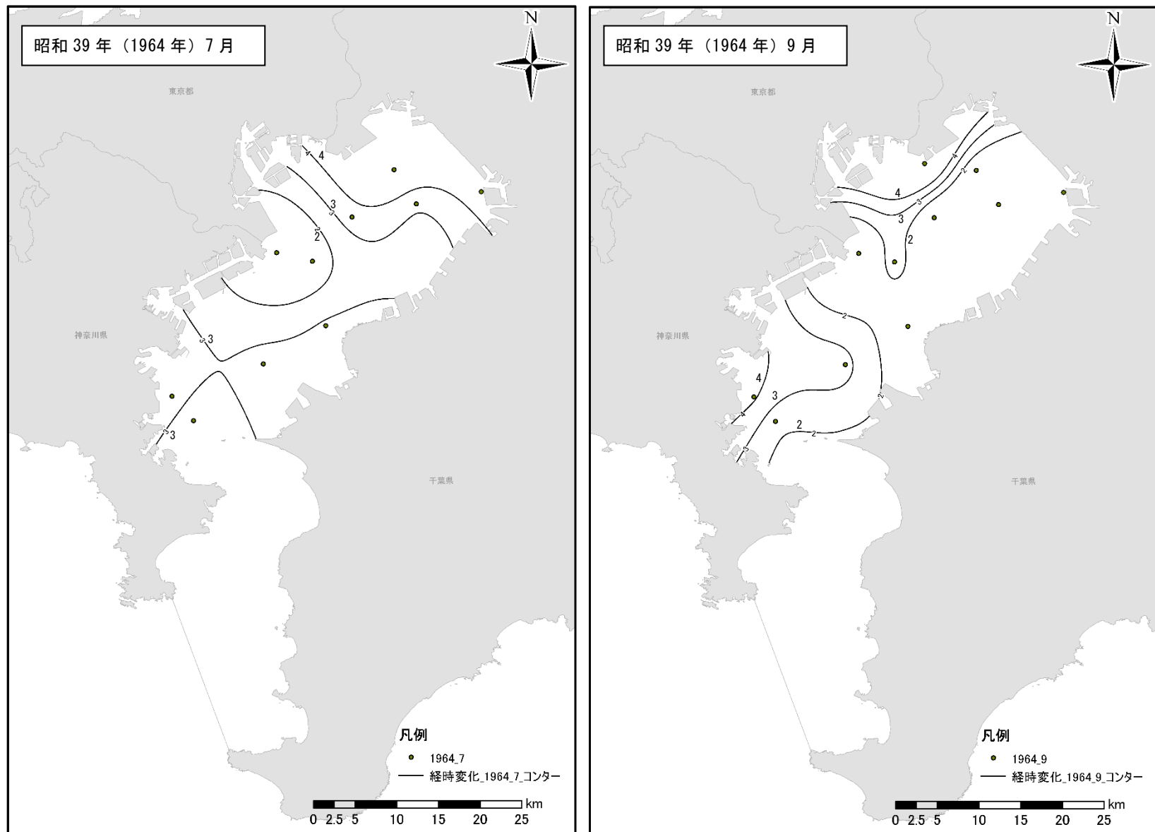
図 1.1.42(10) 昭和30年(1955年)～昭和44年(1969年)の東京湾の底層溶存酸素量の状況
