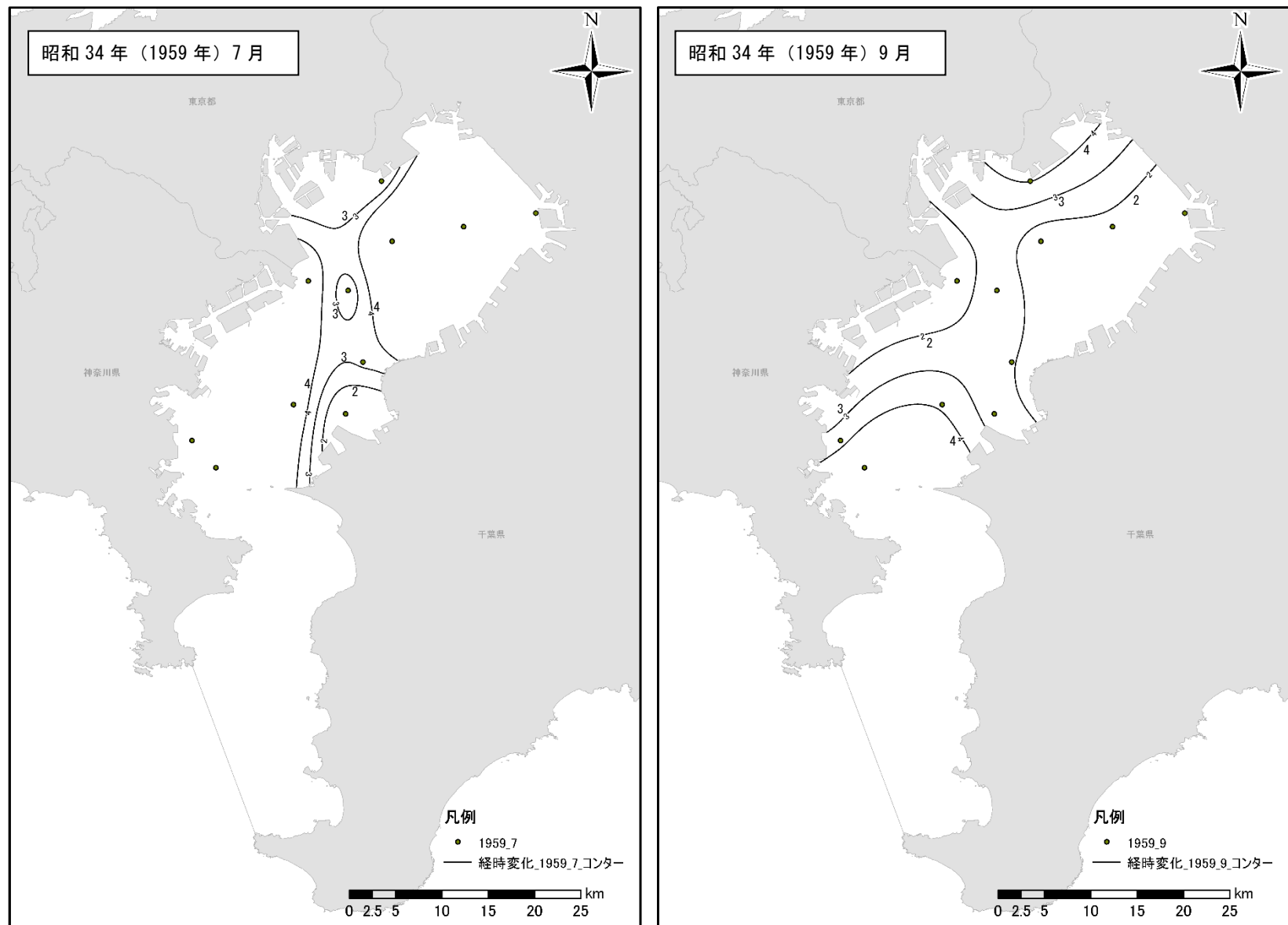
図 1.1.42(5) 昭和30年（1955年）～昭和44年（1969年）の東京湾の底層溶存酸素量の状況
