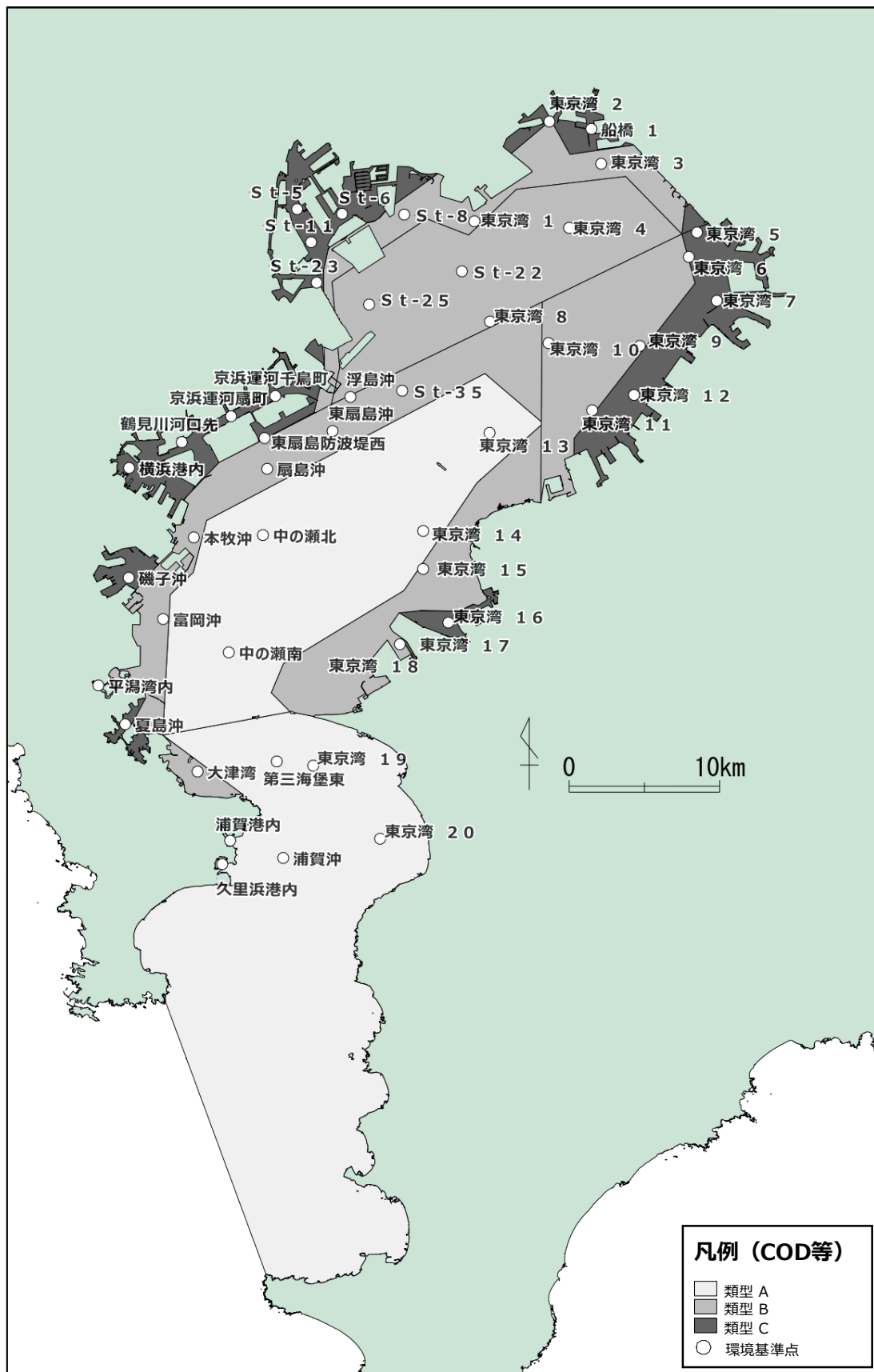
図 1.1.4 水質汚濁に係る環境基準点 (COD)
