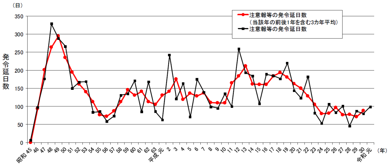
図 2-2-2 光化学オキシダント注意報等の発令遅日数の推移（3年移動平均値）
