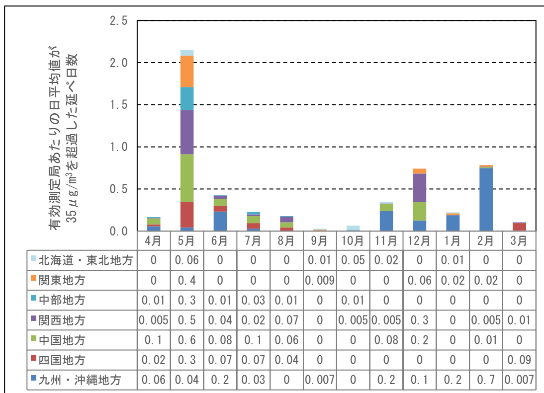
図 1-3-5 令和元年度の各地域における有効測定局当たりの日平均値が 35 \mu\text{g}/\text{m}^3 を超過した延べ日数
