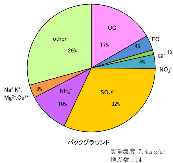
図1 地点分類別の成分割合 (全国)
