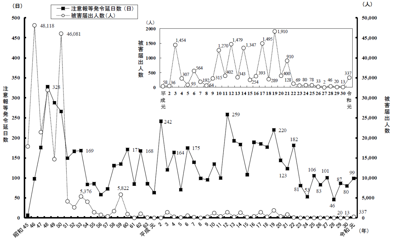
図 2-2-1 光化学オキシダント注意報等の発令遅日数及び被害届出人数の推移
