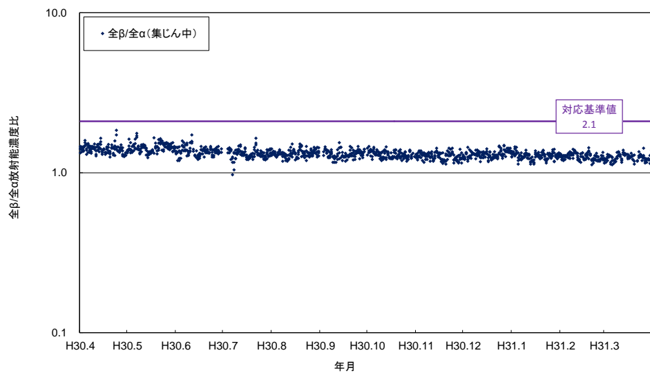
対馬測定所における大気浮遊じん全β/全α放射能濃度比(集じん中)の経時変化
