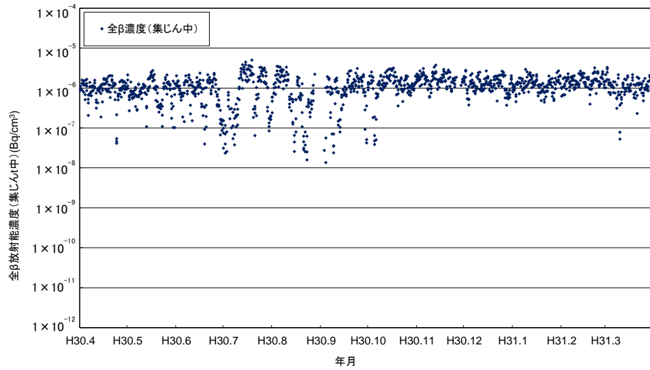
橋原測定所における大気浮遊じん全β放射能濃度(集じん中)の経時変化
