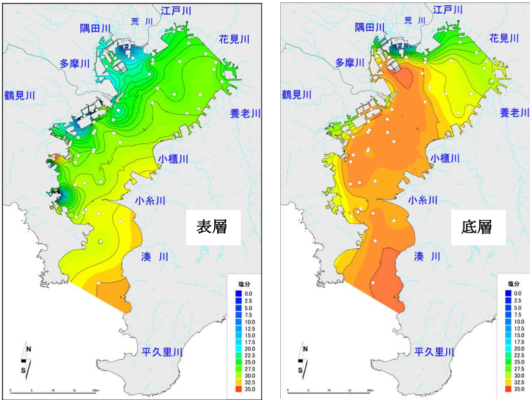
図1-2 塩分の水平分布 (左図：表層、右図：底層)
