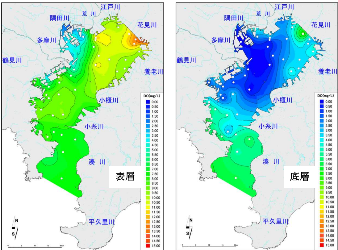
図1-3 DOの水平分布 (左図：表層、右図：底層)
