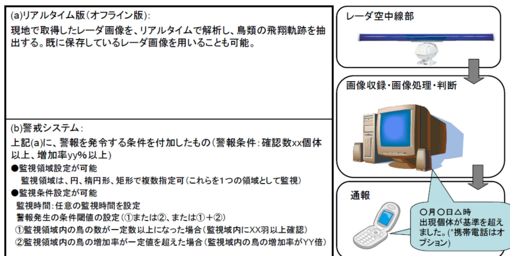
図-21 レーダーによる監視システムの運用管理の例（概要）
