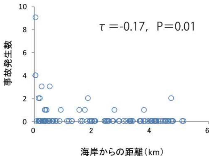
図－４．海ワシ類の風車への衝突事故の件数と各環境要素との関係 (海岸からの距離)
