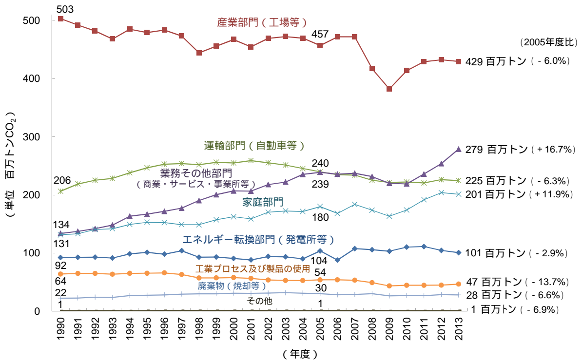
1 図1 我が国における二酸化炭素排出量の部門別の推移 2 (カッコ内の数字は各部門の2013年度排出量の2005年度排出量からの増減率)
