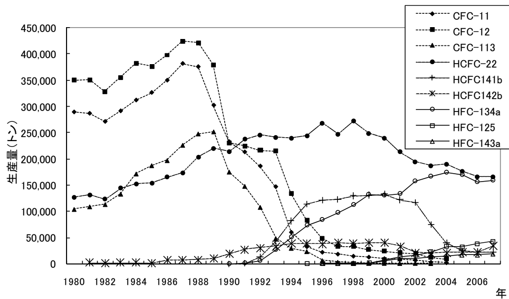
図 4-3 主要なフロン類の年別生産量の推移（1980～2007年） 集計はAFEASに登録のあったデータのみ。単位は重量トン。 （出典）The Alternative Fluorocarbons Environmental Acceptability Study (AFEAS) ウェブサイトより
