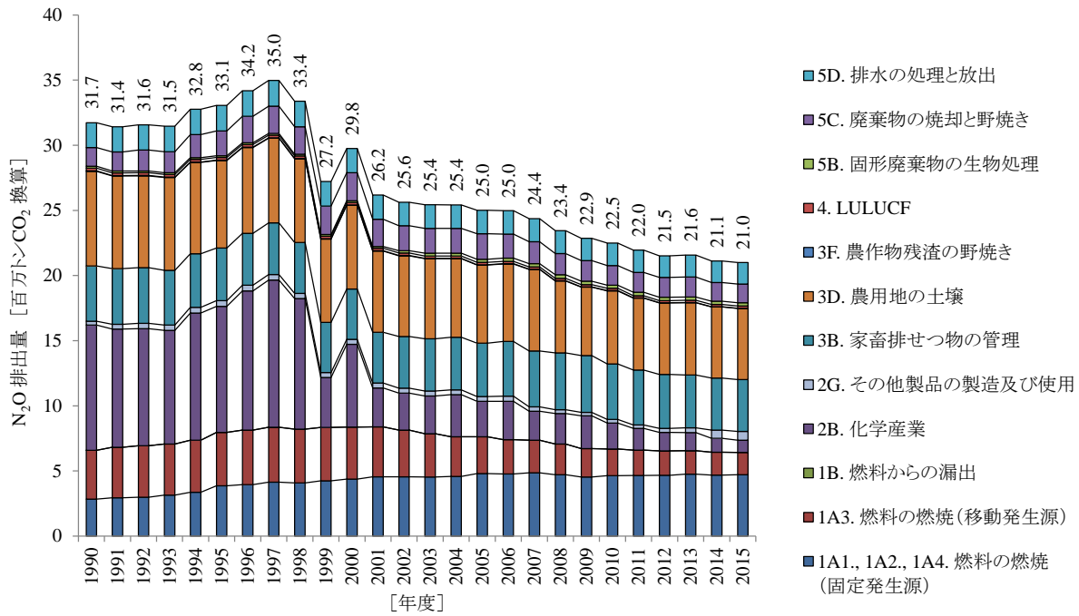
図 2-7 N 2 O 排出量の推移
