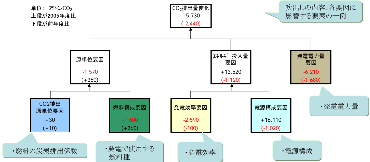
図 2-22 エネルギー転換部門（事業用発電部門）の CO 2 排出量増減要因（電気・熱配分前）（2015 年度）
