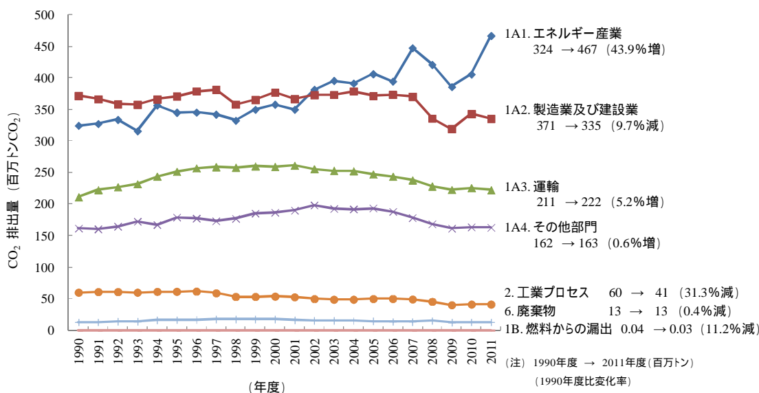
図 2.3 各部門の CO 2 排出量の推移 (かっこ内の数値は1990年度比)
