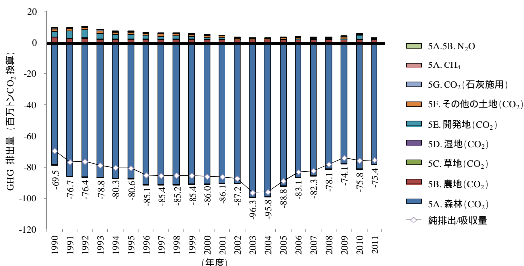
図 2.19 LULUCF 分野からの温室効果ガス排出量及び吸収量の推移
