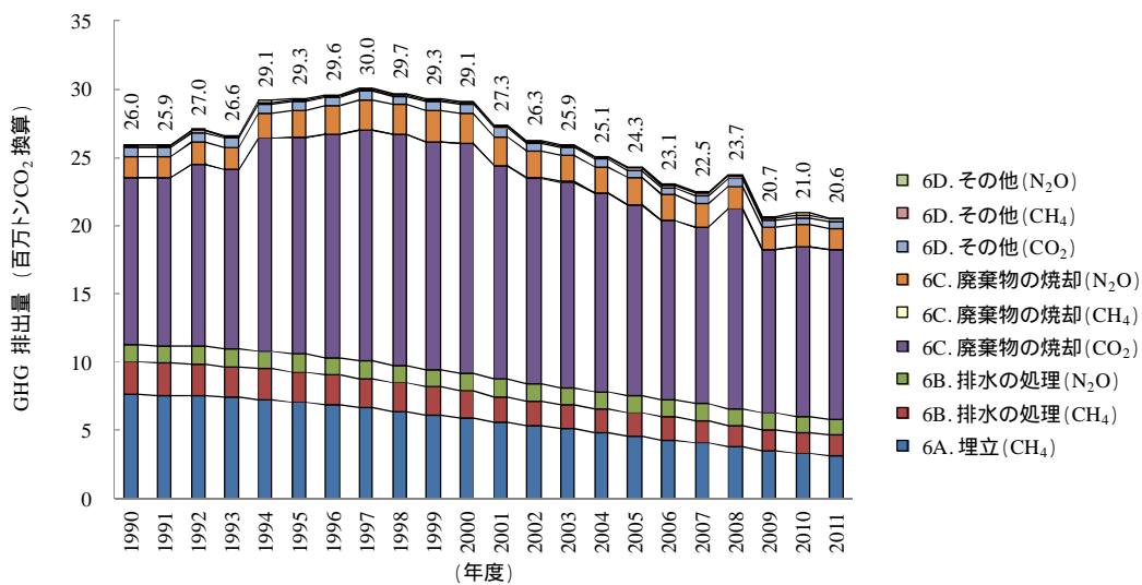
図 2.20 廃棄物分野からの温室効果ガス排出量の推移
