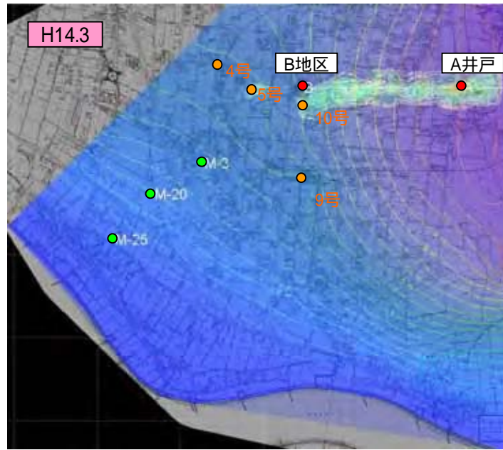
图4.1.2 現況再現解析：深度10m
