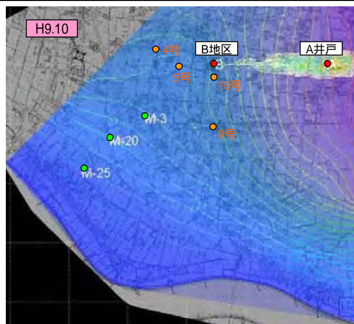
図4.1.2 現況再現解析：深度20m
