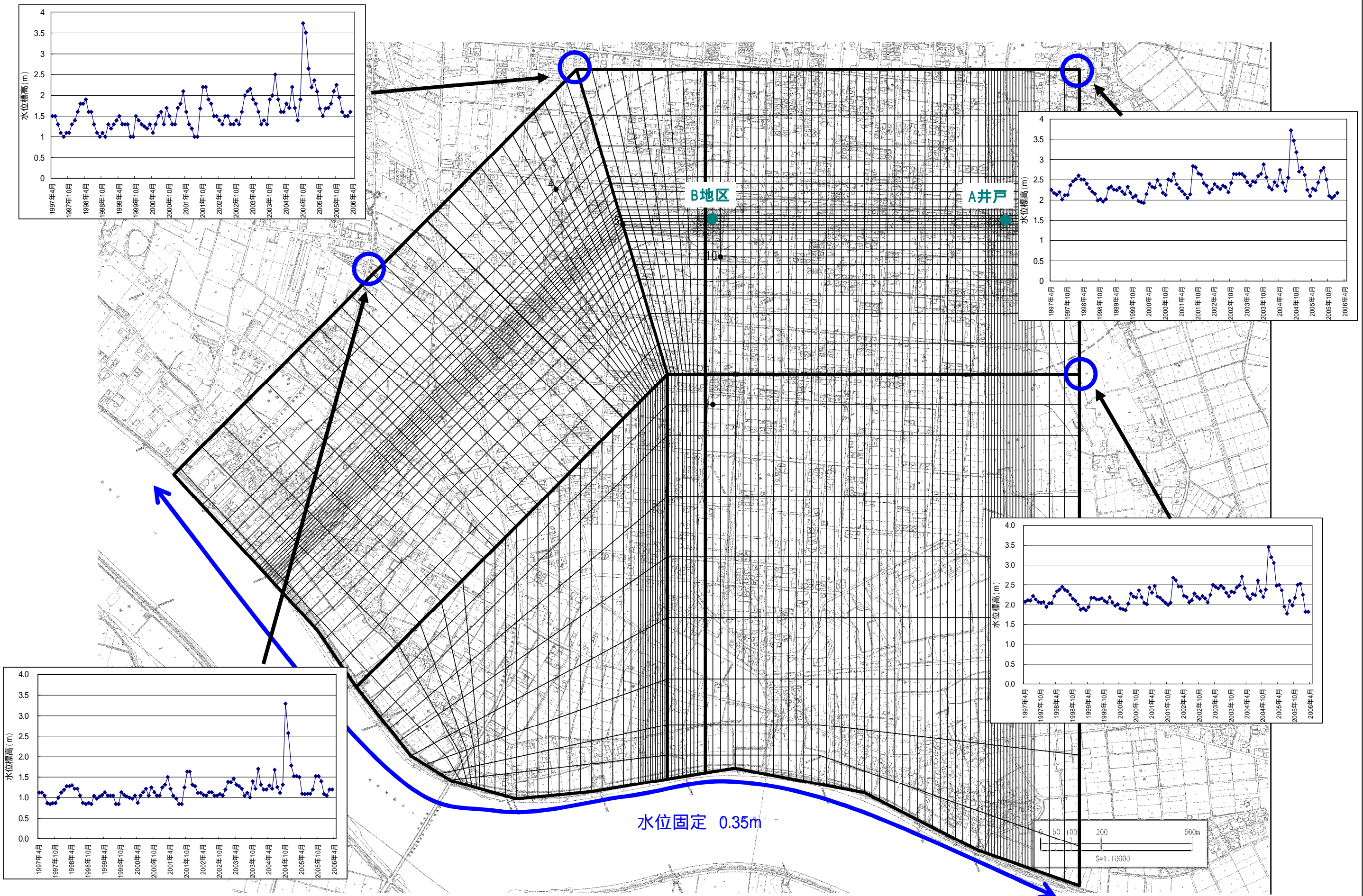
図3.3.1 ABトラック地下水汚染シミュレーション境界条件
