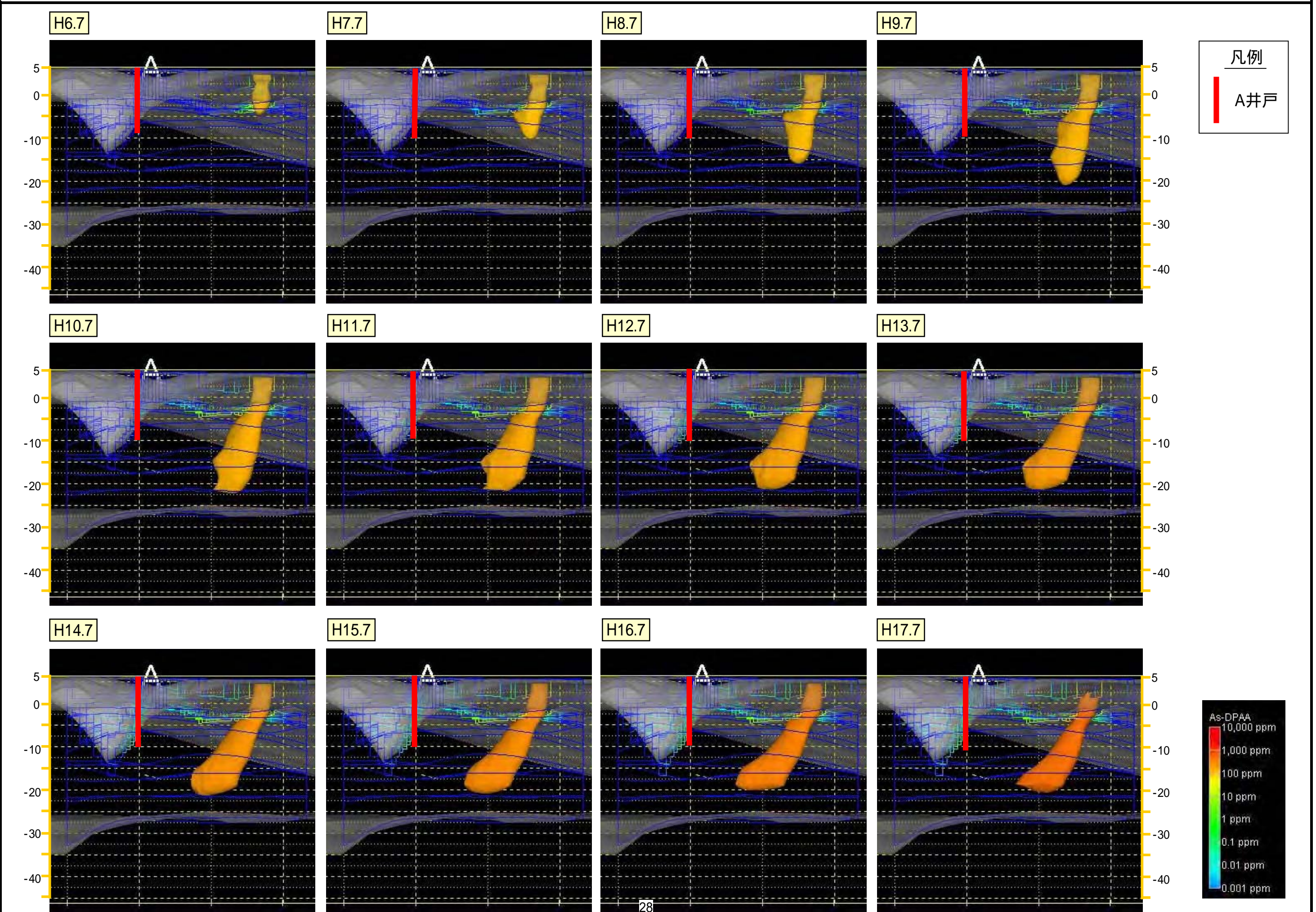
図5.1.6 Case3 初期濃度3,200ppm (ヒ素換算値) 汚染推移 (100ppm)
