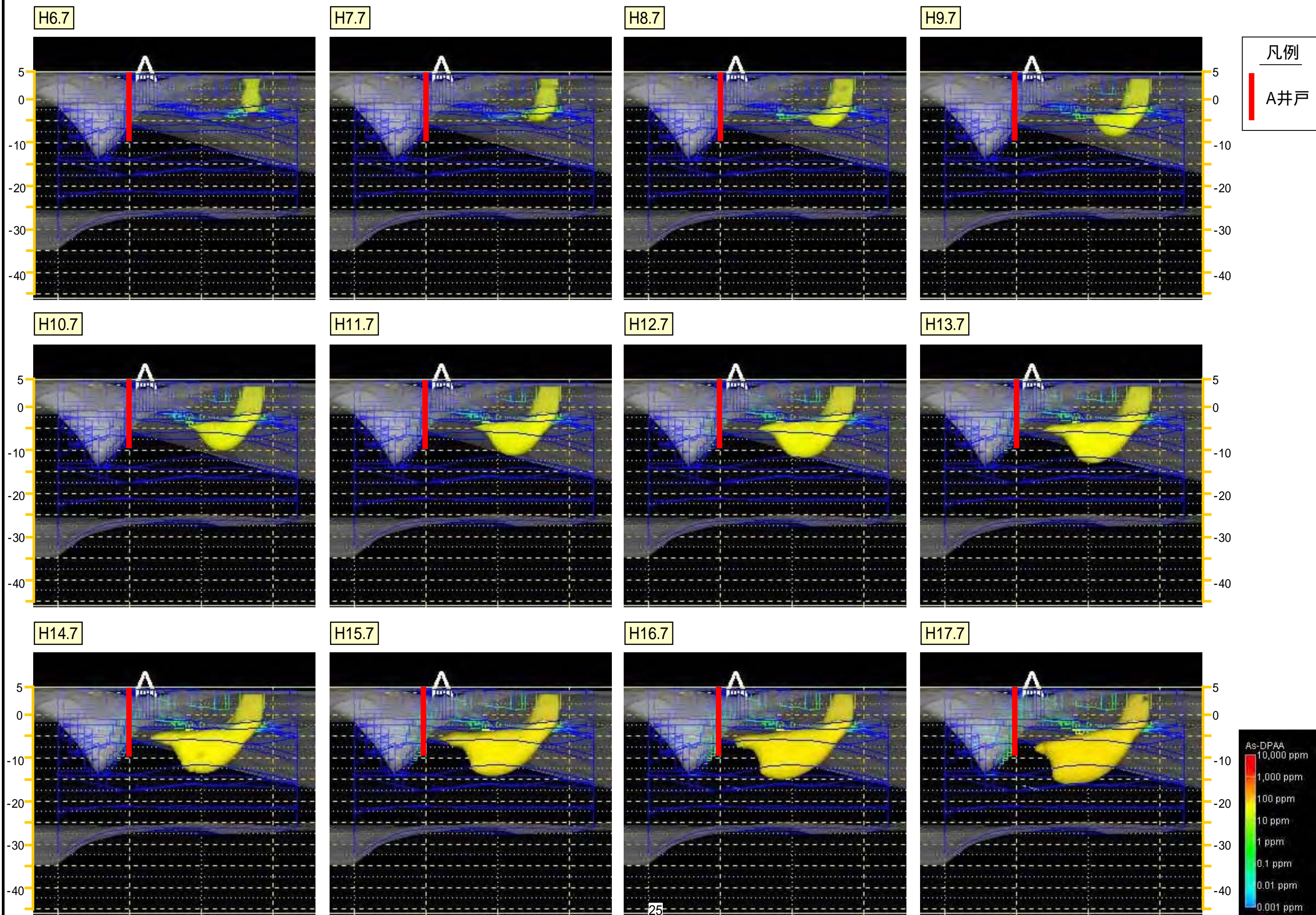
図5.1.4 Case2 初期濃度1,000ppm (ヒ素換算値) 汚染推移 (10ppm)
