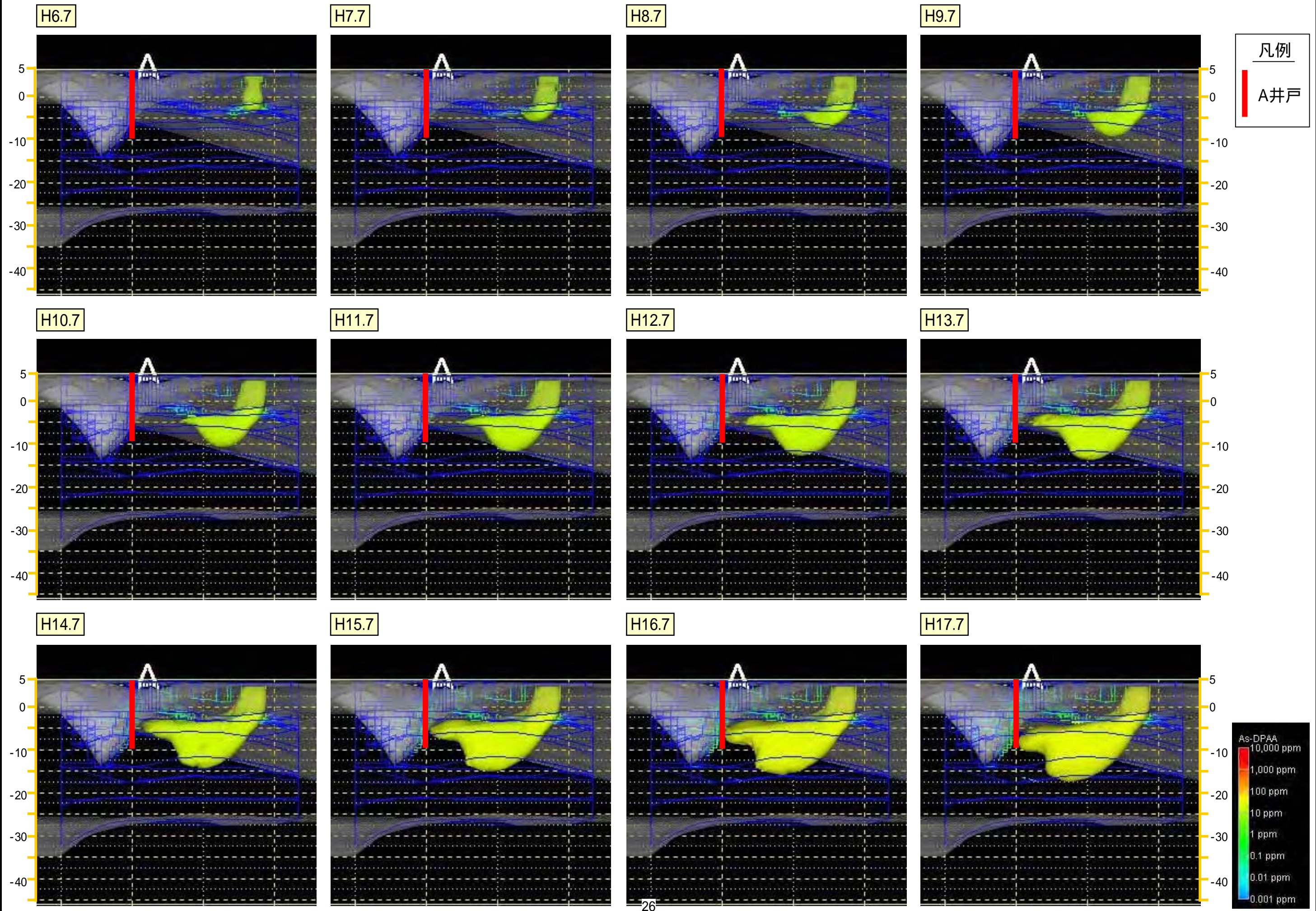
図5.1.4 Case2 初期濃度1,000ppm (ヒ素換算値) 汚染推移 (5ppm)
