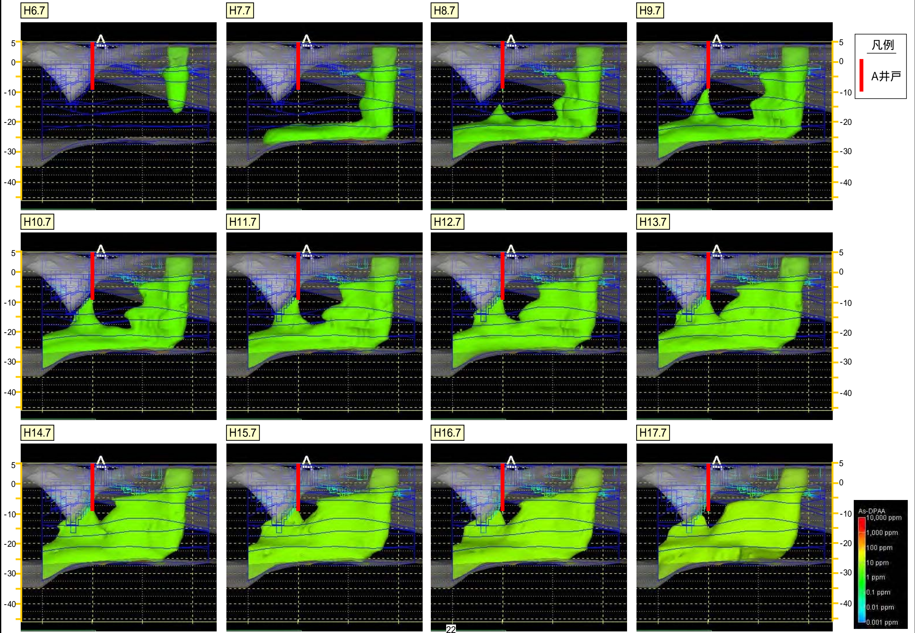
図5.1.2 Case1 初期濃度10,000ppm (ヒ素換算値) 汚染推移 (5ppm)
