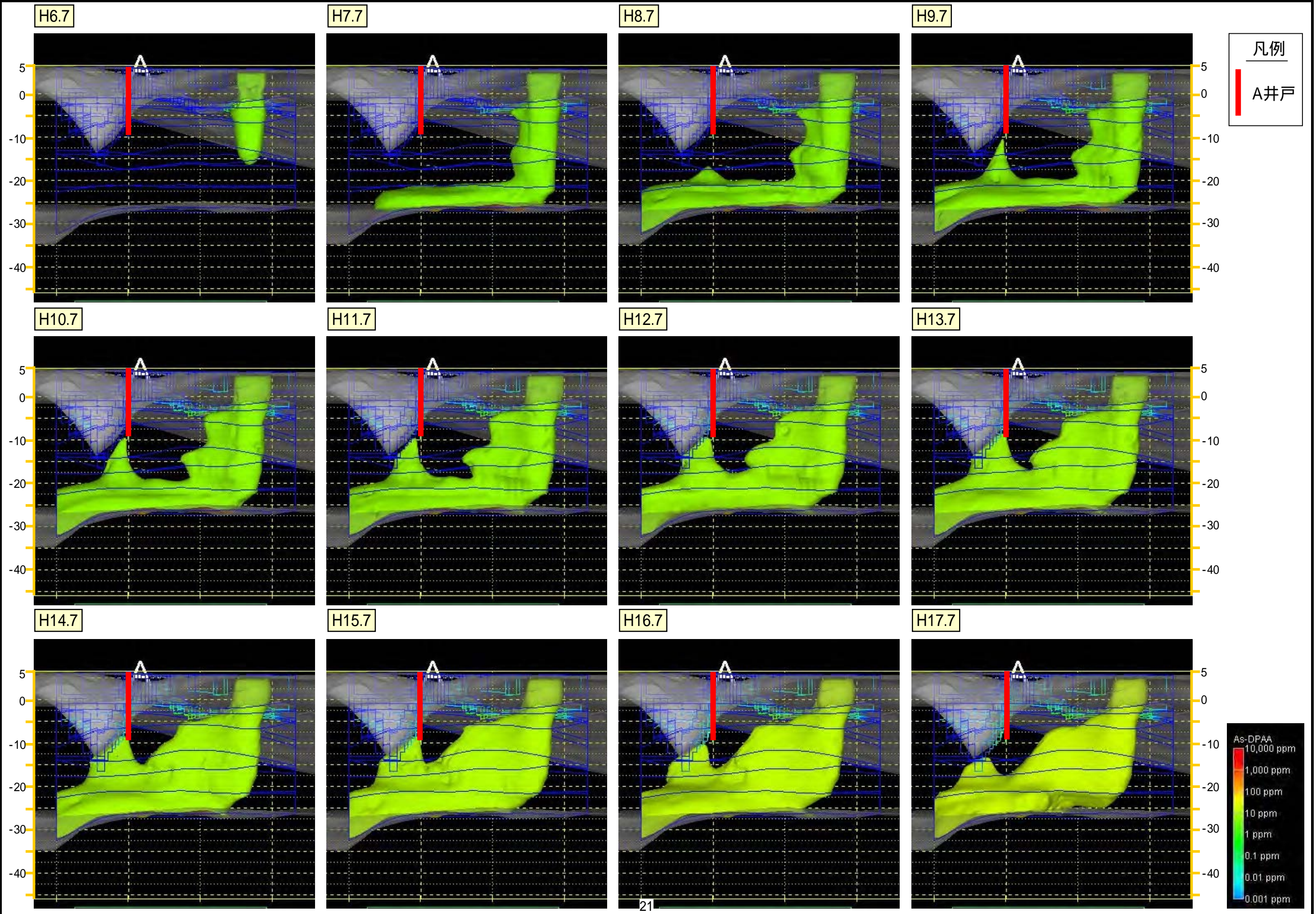
図5.1.2 Case1 初期濃度10,000ppm (ヒ素換算値) 汚染推移 (10ppm)
