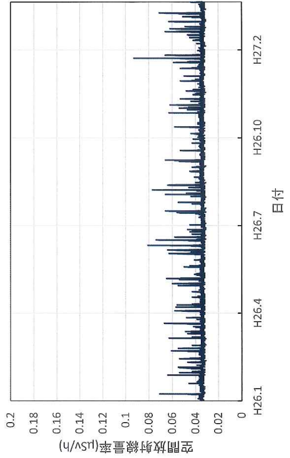
熊本県荒尾市 荒尾市役所の空間放射線量率(10分値使用)
