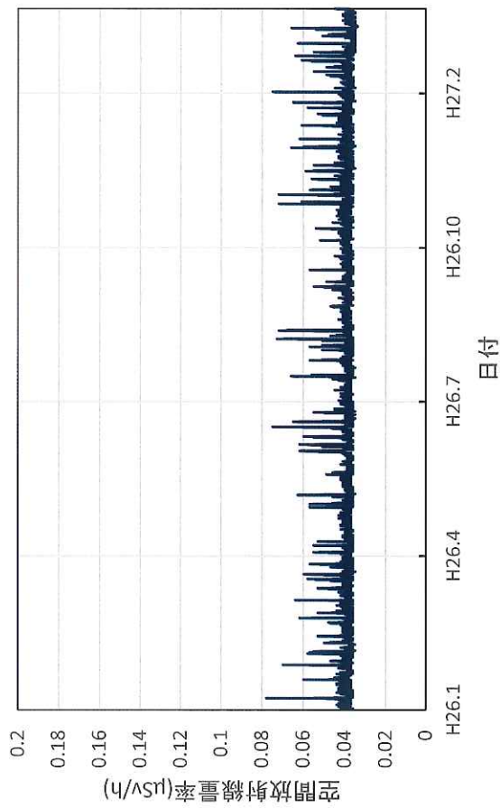
大分県日田市 日田総合庁舎の空間放射線量率(10分値使用)
