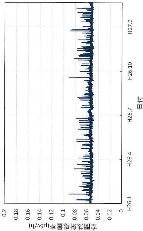
愛媛県八幡浜市 市立武道館の空間放射線量率(10分値使用)
