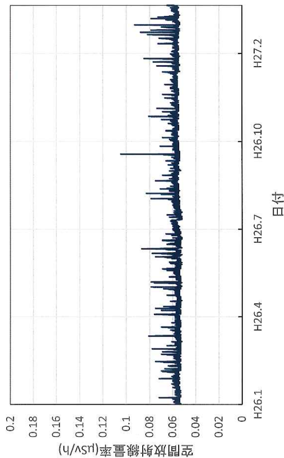
宮崎県延岡市 延岡保健所の空間放射線量率(10分値使用)
