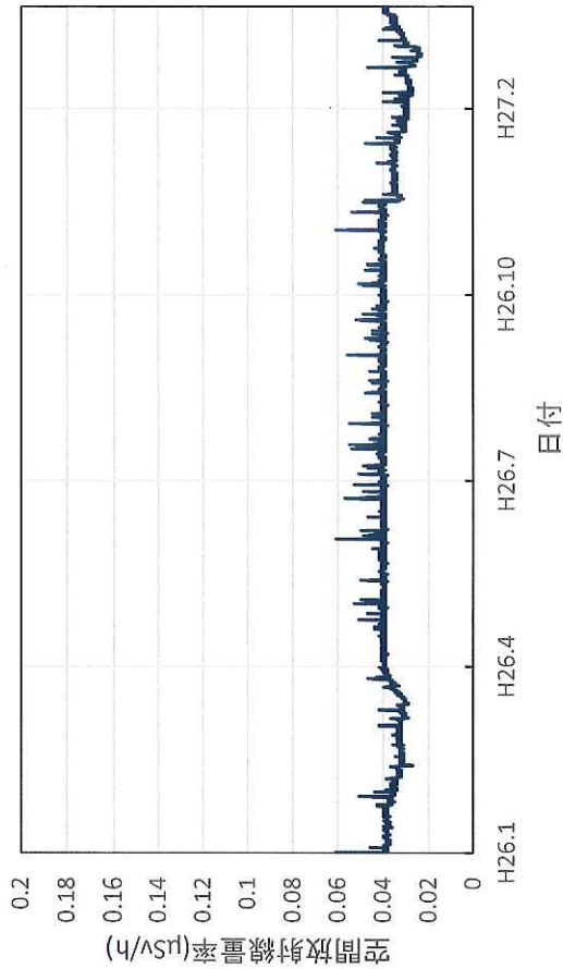
北海道釧路市 釧路総合振興局の空間放射線量率(10分値使用)
