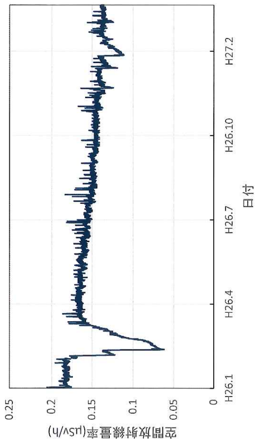
福島県二本松市 県男女共生センターの空間放射線量率(10分 値使用)
