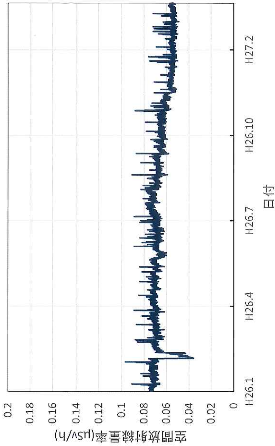
茨城県龍ヶ崎市 龍ヶ崎市役所の空間放射線量率(10分値使用)
