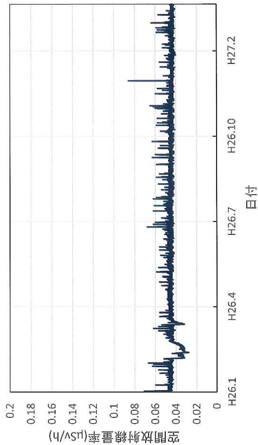
岩手県釜石市 釜石地区合同庁舎の空間放射線量率(10分値使用)
