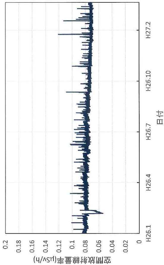
茨城県水戸市 茨城県庁の空間放射線量率(10分値使用)
