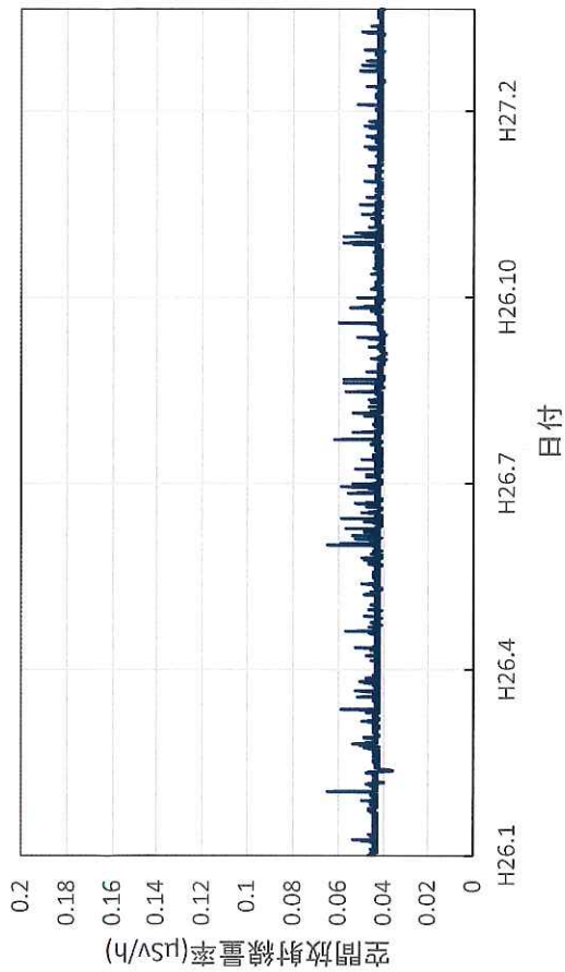
栃木県宇都宮市 県保健環境センターの空間放射線量率(10分値 値使用)
