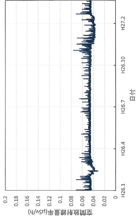
山形県山形市 県衛生研究所の空間放射線量率(10分値使用)
