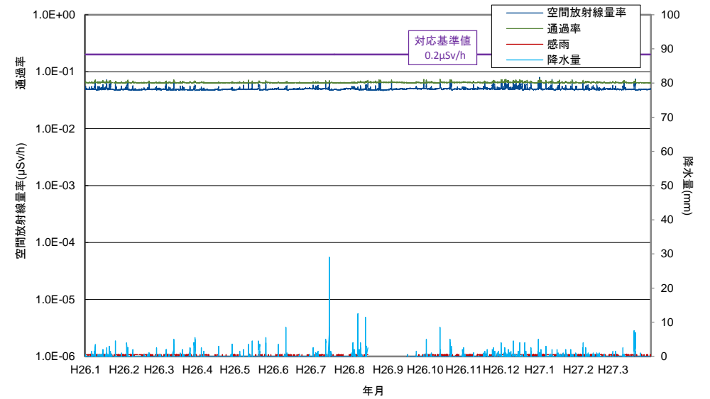
付図3-5 隠岐測定所における空間放射線量率、通過率及び降水量の経時変化 (H26年1月～H27年3月)
