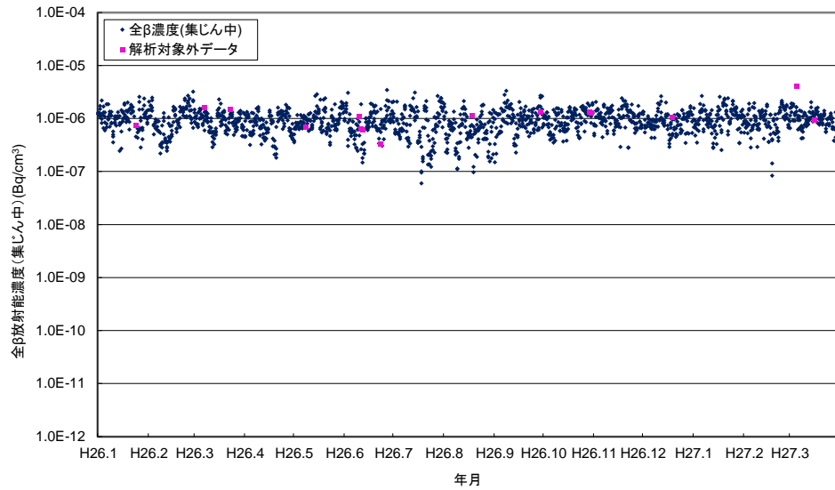
付図4-23 隠岐測定所における大気浮遊じんの大β放射能濃度(集jin中)の経時変化
