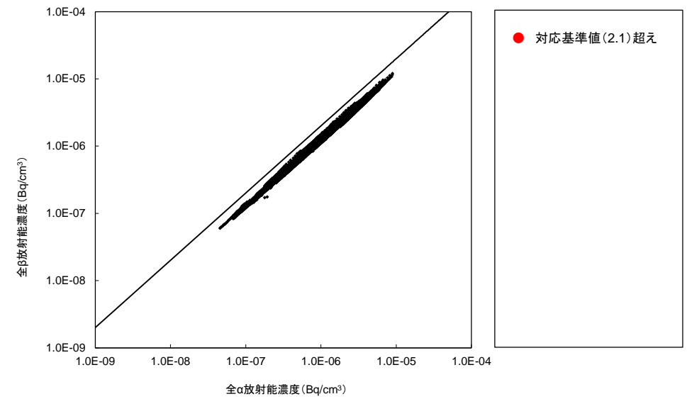
隠岐測定所における全α及び全β放射能濃度分布 (集jin開始後40分以上の測定データを採用)
