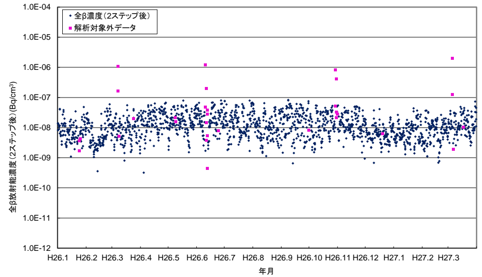
付図4-24 隠岐測定所における大気浮遊じんの大β放射能濃度(2ステップ後)の経時変化
