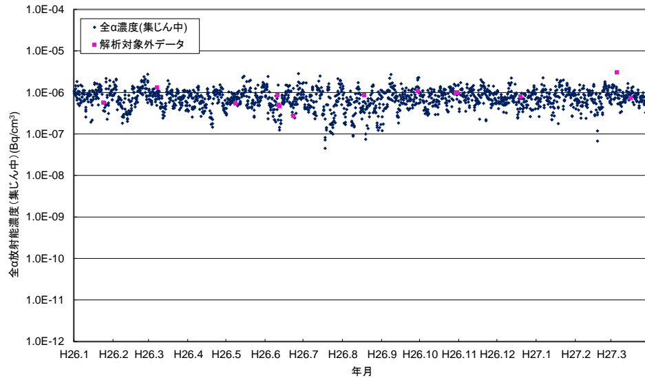
付図4-21 隠岐測定所における大気浮遊じんの大α放射能濃度 (集じん中) の経時変化
