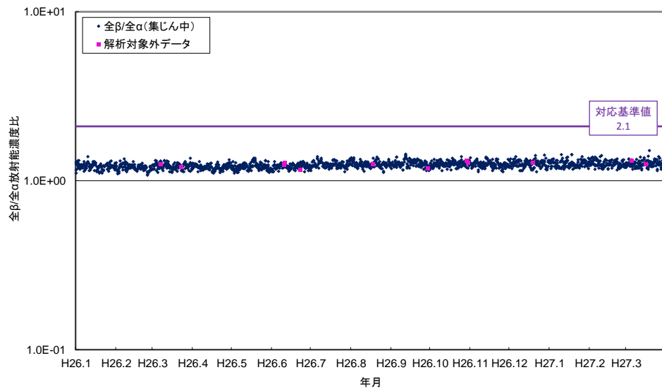
付図4-25 隠岐測定所における大気浮遊じんの大β/全α放射能濃度比(集jin中)の経時変化
