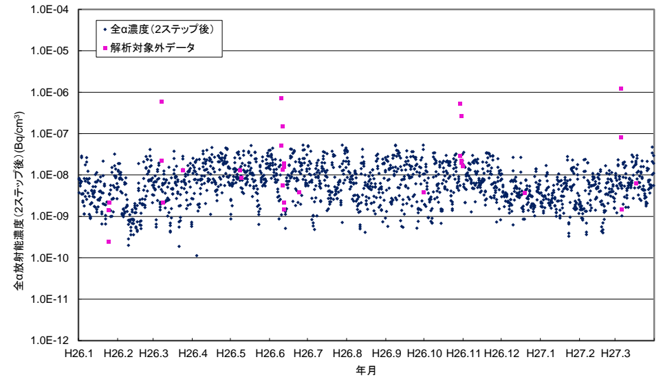
付図4-22 隠岐測定所における大気浮遊じんの大α放射能濃度 (2ステップ後) の経時変化
