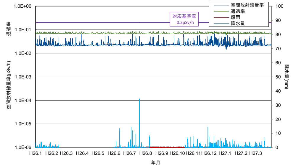
付図3-4 越前岬測定所における空間放射線量率、通過率及び降水量の経時変化 (H26年1月～H27年3月)
