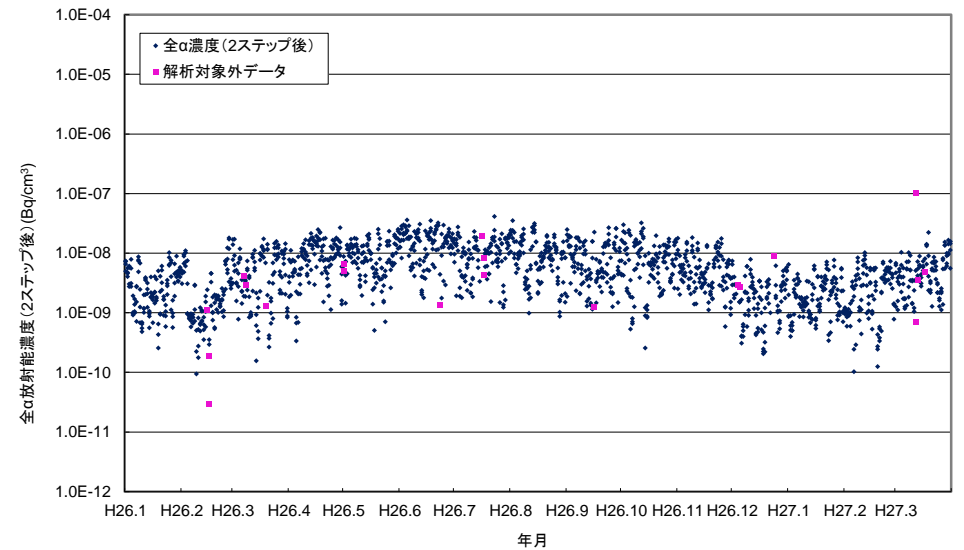
付図4-17 越前岬測定所における大気浮遊じんの全α放射能濃度(2ステップ後)の経時変化
