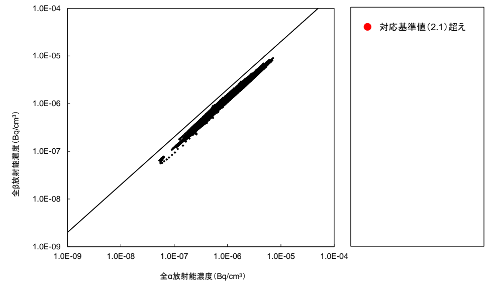
佐渡関岬測定所に全α及び全β放射能濃度分布 (集じん開始後40分以上の測定データを採用)
