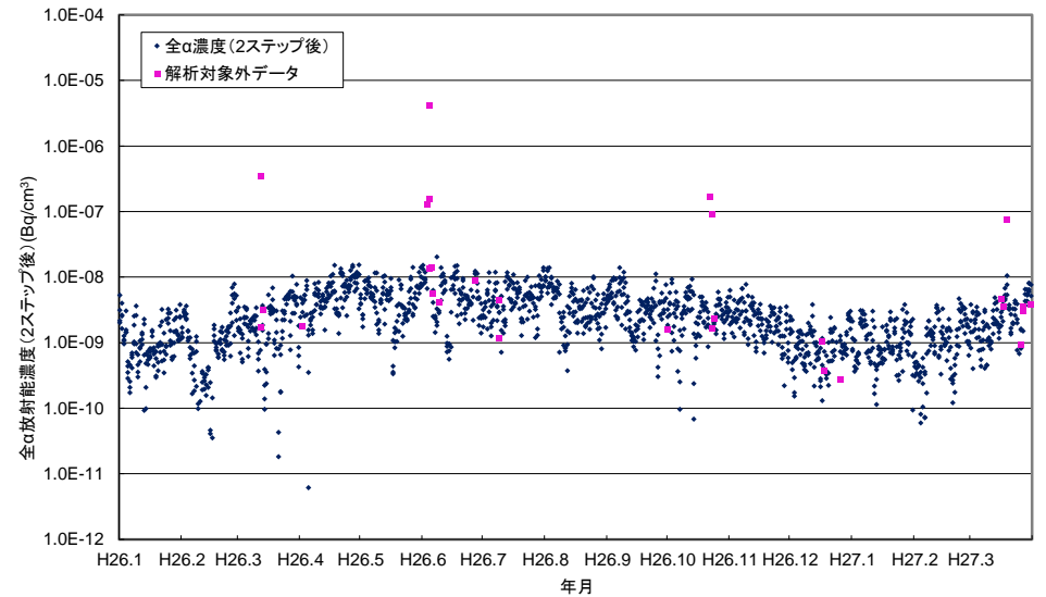
付図4-12 佐渡関岬測定所における大気浮遊じんの全α放射能濃度(2ステップ後)の経時変化
