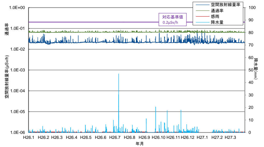
付図3-3 佐渡関岬測定所における空間放射線量率、通過率及び降水量の経時変化 (H26年1月～H27年3月)
