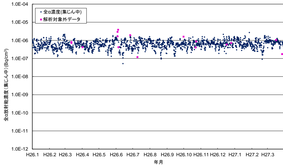
付図4-11 佐渡関岬測定所における大気浮遊じんの全α放射能濃度(集じん中)の経時変化
