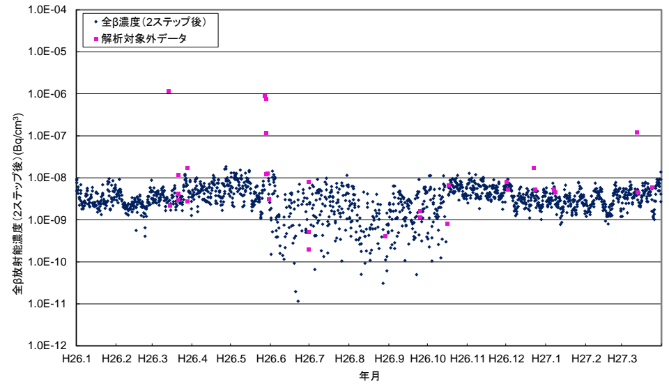
付図4-9 竜飛岬測定所における大気浮遊じんの全β放射能濃度(2ステップ後)の経時変化
