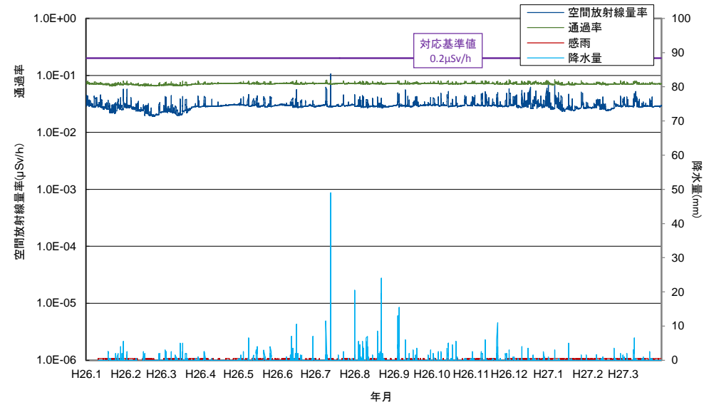
付図3-2 竜飛岬測定所における空間放射線量率、通過率及び降水量の経時変化(H26年1月～H27年3月)
