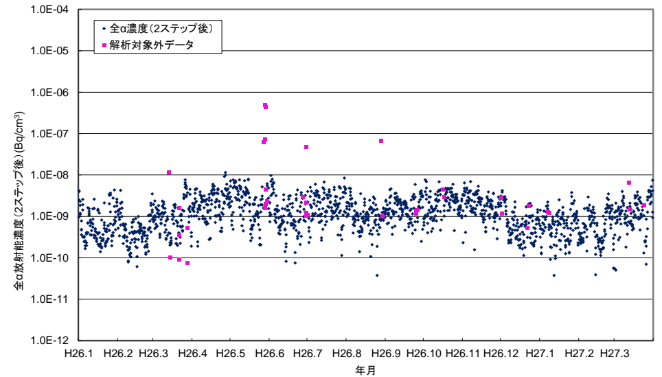
付図4-7 竜飛岬測定所における大気浮遊じんの全α放射能濃度(2ステップ後)の経時変化
