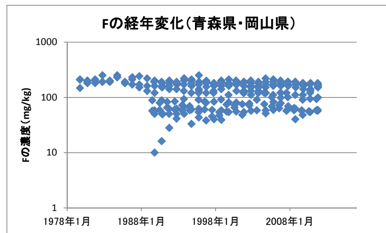
図 2-8-1 F の検出状況の経年変化
