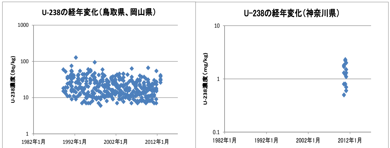
図 2-17-1 U-238 の検出状況の経年変化
