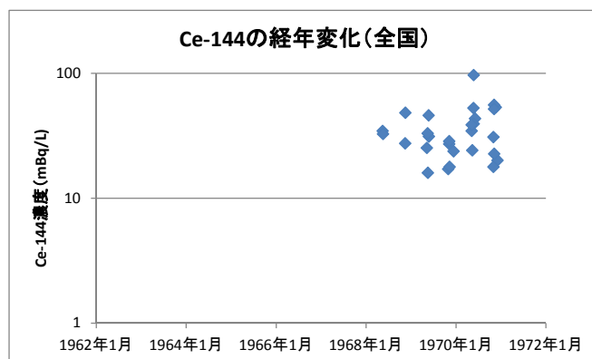
図 2-4-1 Ce-144 の検出状況の経年変化
