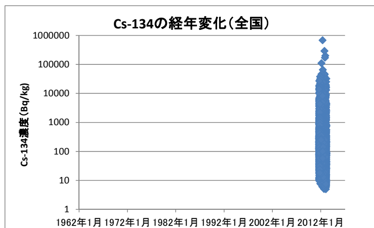
図 2-6-1 Cs-134 の検出状況の経年変化
