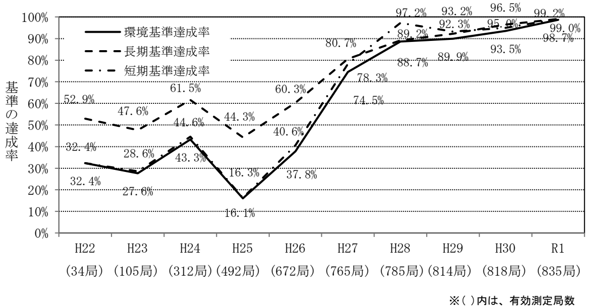
図7-2-2 長期基準及び短期基準達成状況の推移
