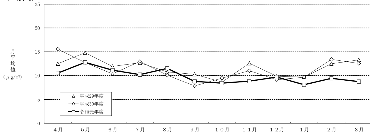
図7-2-18 微小粒子状物質の月平均値の推移
