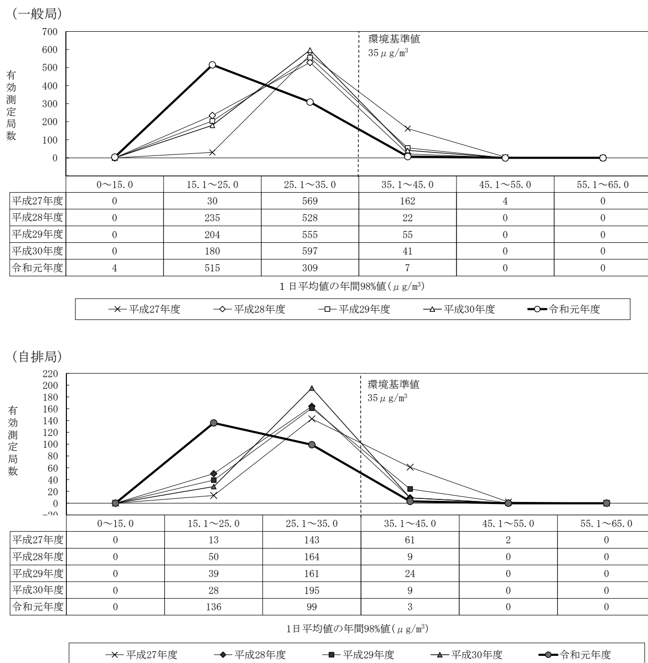
図7-2-16 1日平均値の年間98パーセンタイル値の濃度範囲別測定局数
