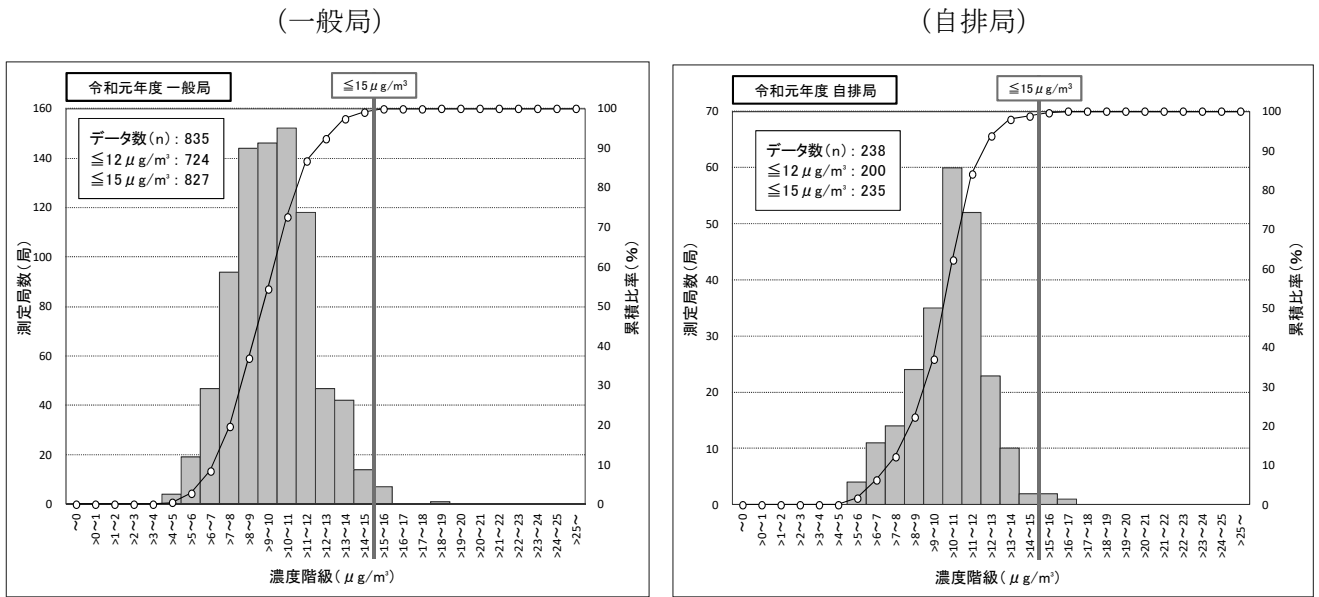
図7-2-4 年平均値のヒストグラム
