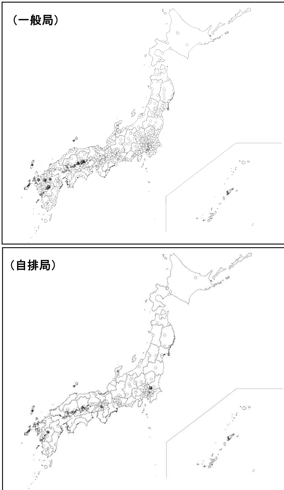
図7-2-11 長期基準及び短期基準達成状況（全国）
