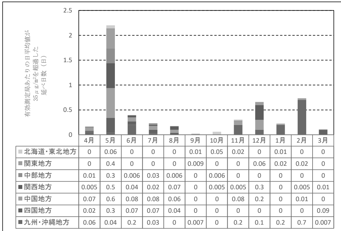
図7-2-9 月別・地域別の日平均値が 35 \mu\text{g}/\text{m}^3 を超過した延べ日数（有効測定局あたり）（令和元年度）
