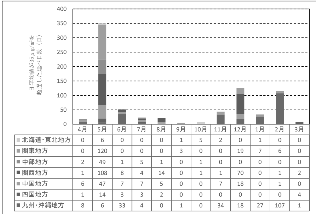
図7-2-8 月別・地域別の日平均値が 35 \mu\text{g}/\text{m}^3 を超過した延べ日数（令和元年度）
