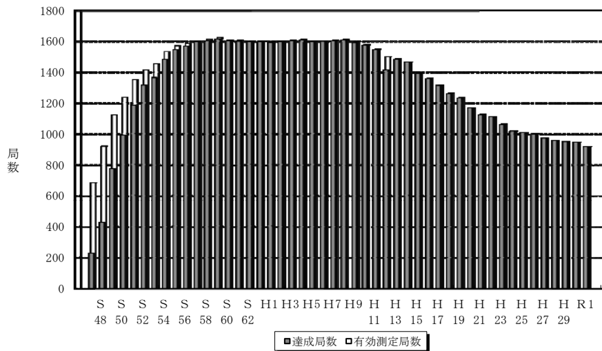
図5-2-1 環境基準達成状況
