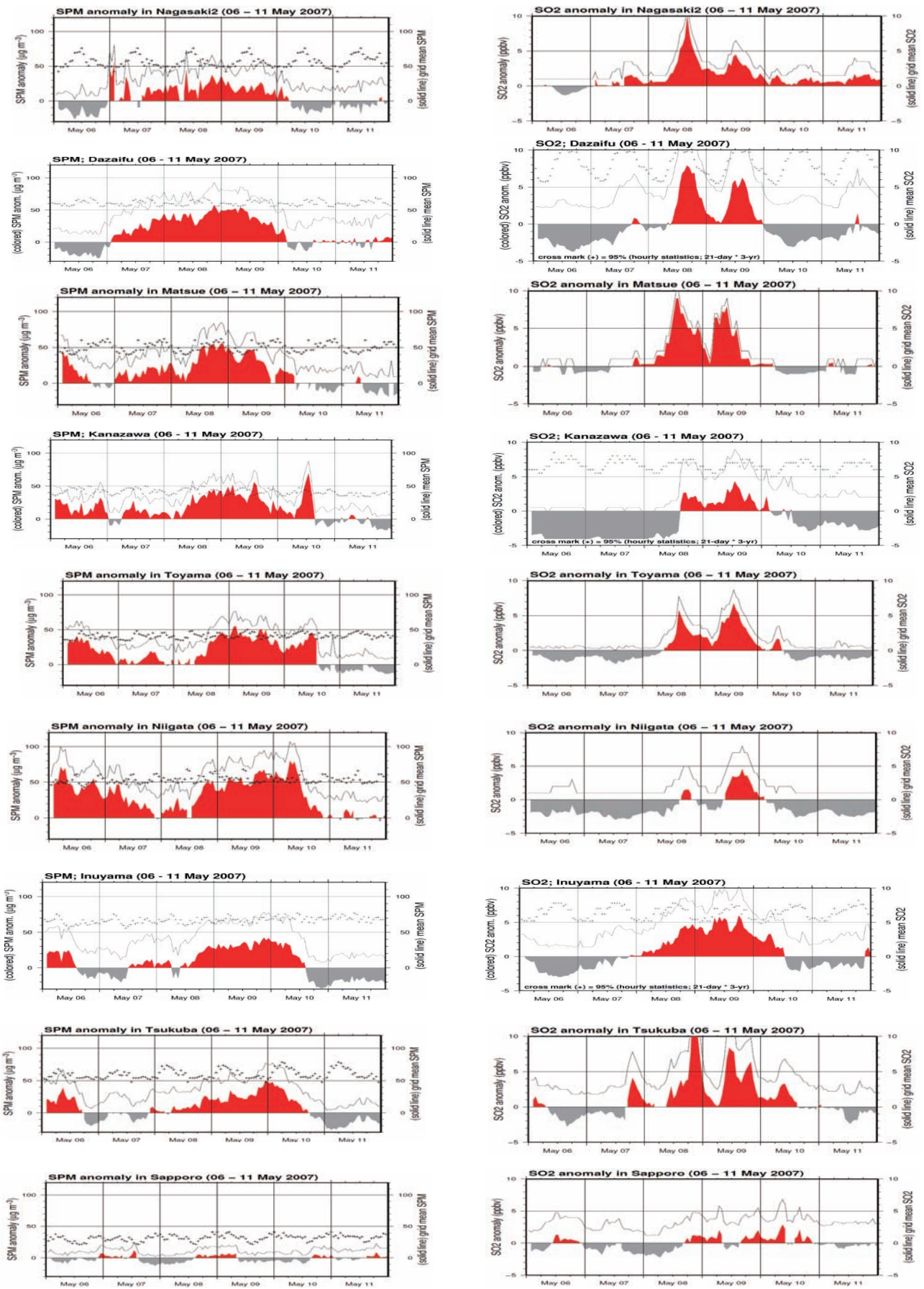
図 7-4 SPM(左列), SO 2 (右列) 格子平均(実線)および偏差(カラー; 正偏差を赤, 負偏差をグレー)の時系列変化(イベント1). SPMの図中にある+マークは, 近年3年間(2004-2006年)の対象日とその前後10日間の時刻別格子平均値に関する95パーセント値
