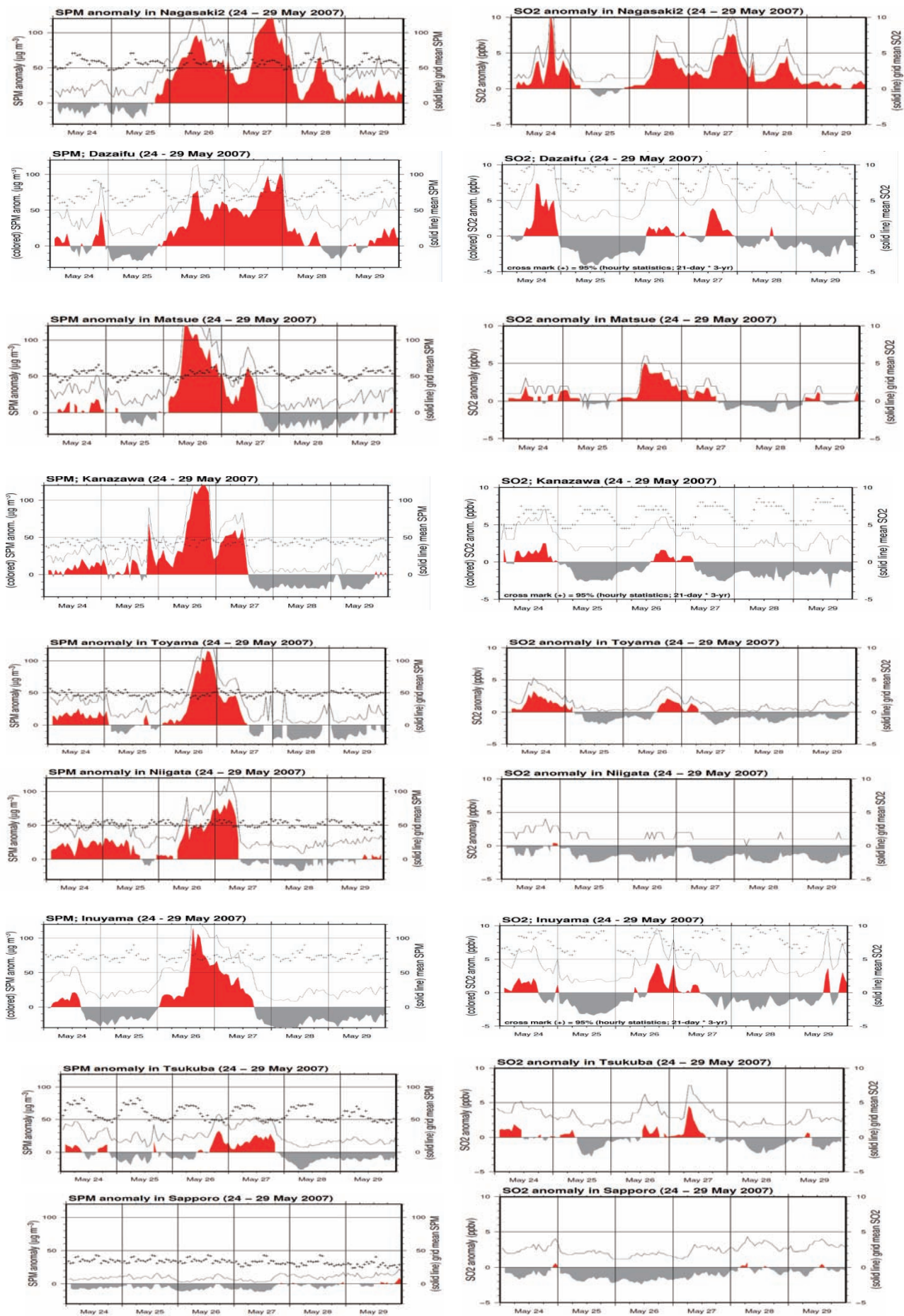
図 7-5 SPM(左列), SO 2 (右列) 格子平均(実線)および偏差(カラー; 正偏差を赤, 負偏差をグレー)の時系列変化(イベント1)。SPMの図中にある+マークは、近年3年間(2004-2006年)の対象日とその前後10日間の時刻別格子平均値に関する95パーセンタイル値
