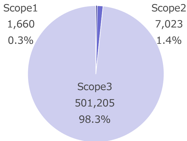
● Scope別CO 2 排出量 (t-CO 2 )
