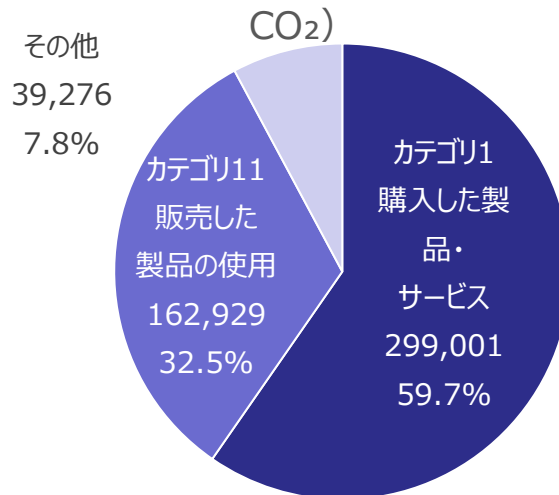
● Scope3 カテゴリ別CO 2 排出量 (t-CO 2 )
